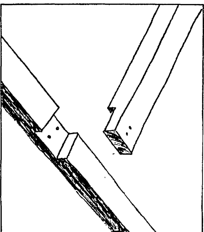
Unión de soleras en "T"
