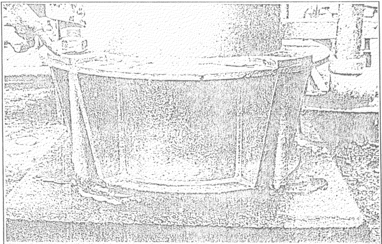
Fotografía N° 7 - Pernos fallados a tracción en la torre GV - 420
