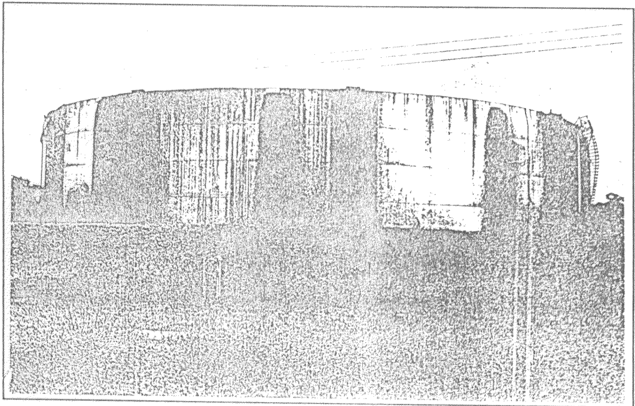
Fotografía N°10 - Daños en el tanque T - 705 para almacenamiento de crudo. Derrames por el nivel de techo
