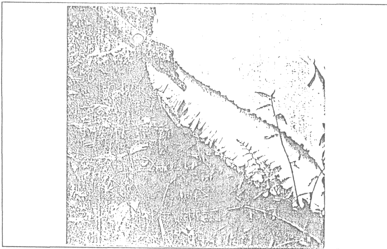
Fotografía N° 12 - Falla por pandeo en tanque T - 745
