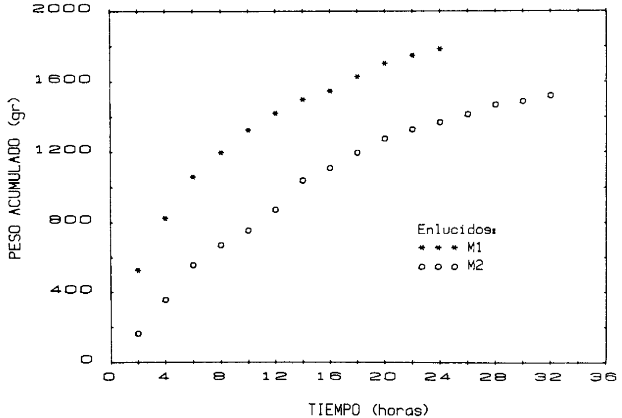
Figura 3.2 Pérdida Acumulada de Material vs. Tiempo (Ensayo de Enlucidos Aplicados sobre Muretes) Enlucidos M1 y M2
