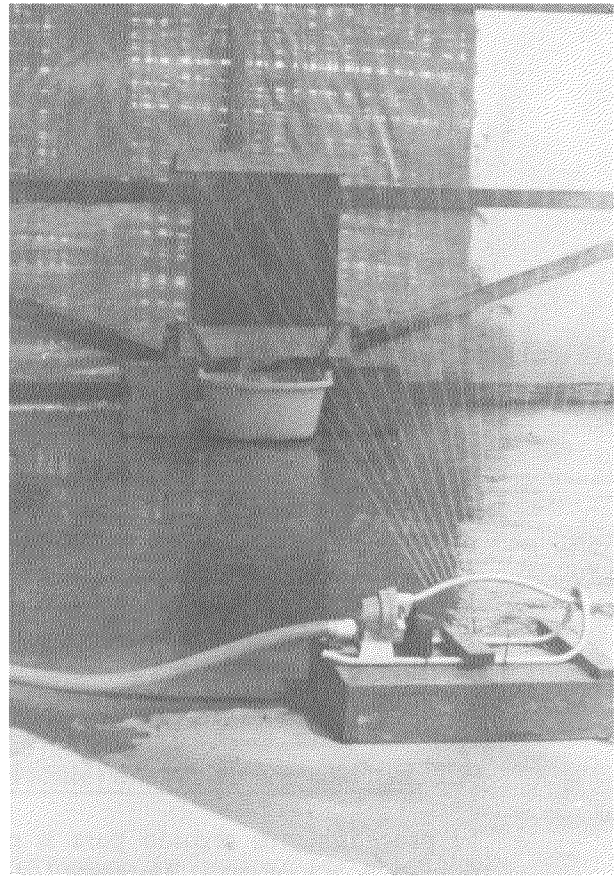
Fig. 3.1 Dispositivo de Ensayo (Enlucidos Aplicados sobre Muretes)
