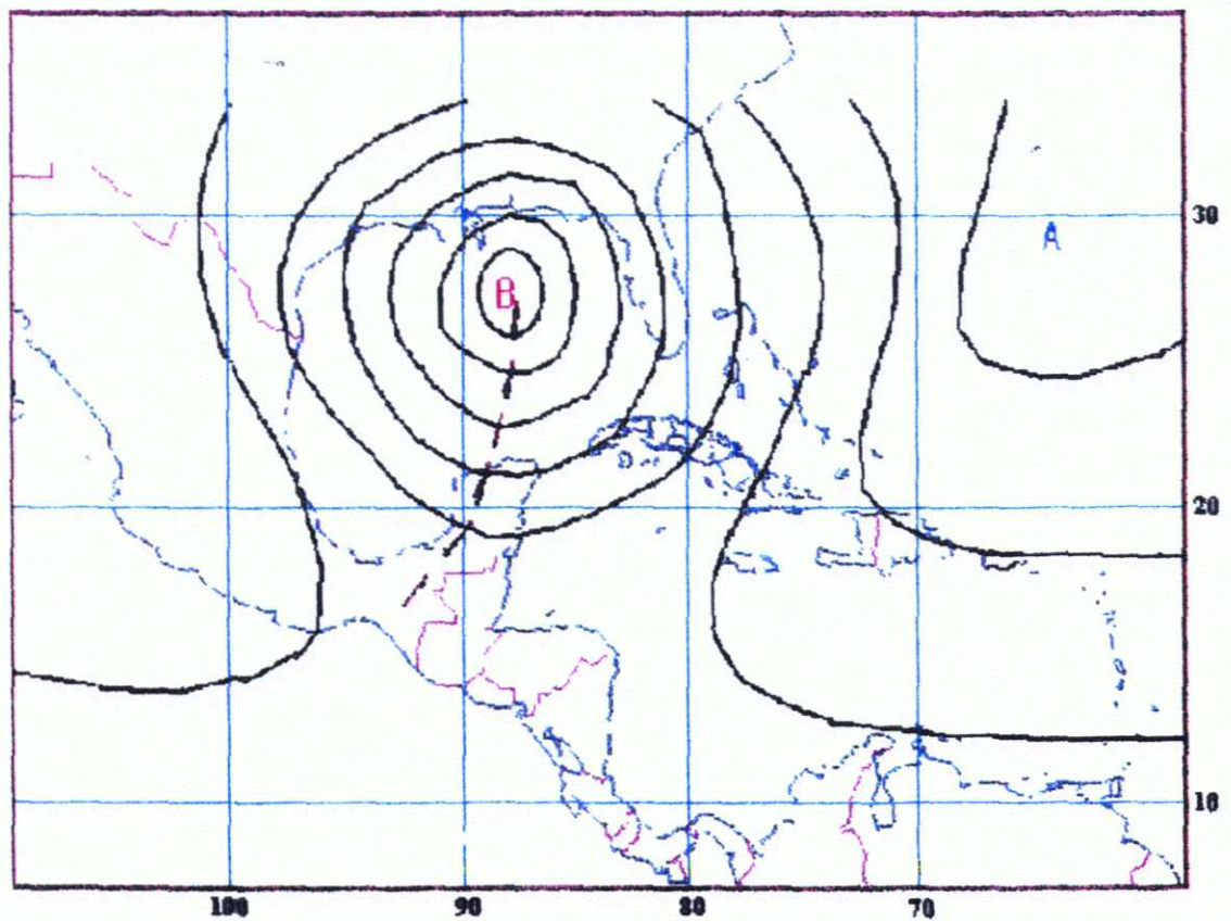
Figura 1.2.2 Tipo sinóptico 2 para inundaciones costeras
