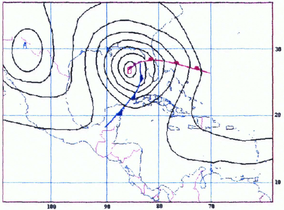
Figura 1.2.1 Tipo sinóptico 1 para inundaciones costeras
