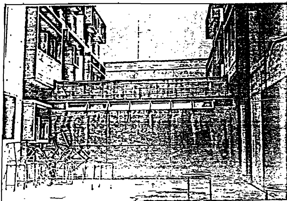
Foto N°20 ESTRUCTURA ENTRE LOS CUERPOS A3 y A4 (SUR)
