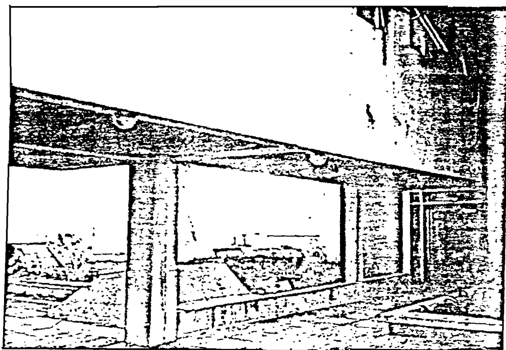
Foto N°8 PASILLO DE COMUNICACION ENTRE LA TORRE Y EL CUERPO C.
