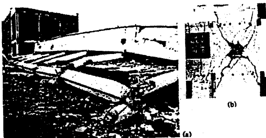
Fig. 1 Falla de uniones viga-columna en (a) el sismo de El Asnam y (b) en un espécimen de laboratorio
