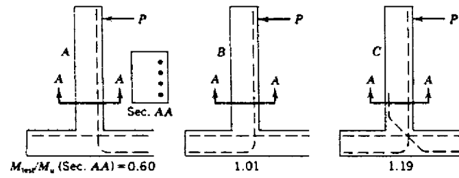
Fig. 13 Uniones en "T"
