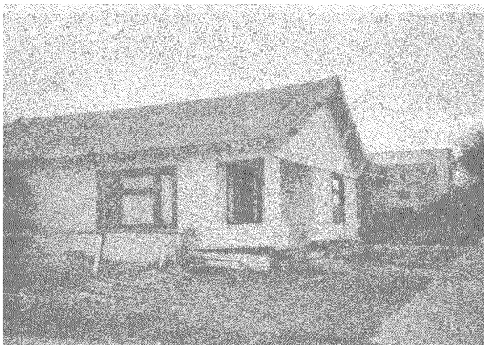
FOTO 5.7: DAÑOS EN LOS APOYOS DE MADERA, WATSONVILLE
