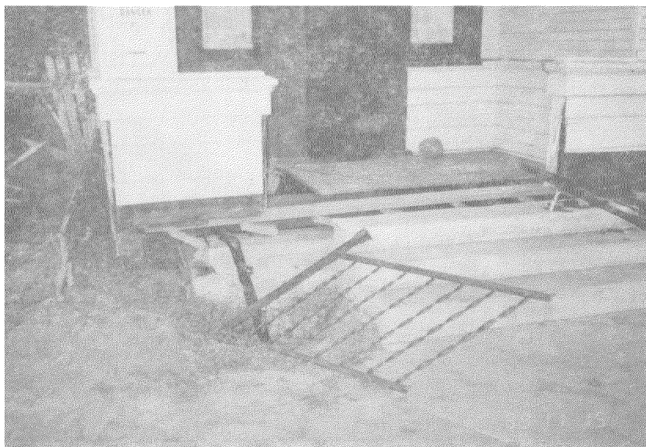
FOTO 5.8: DAÑOS EN LOS APOYOS DE MADERA WATSONVILLE
