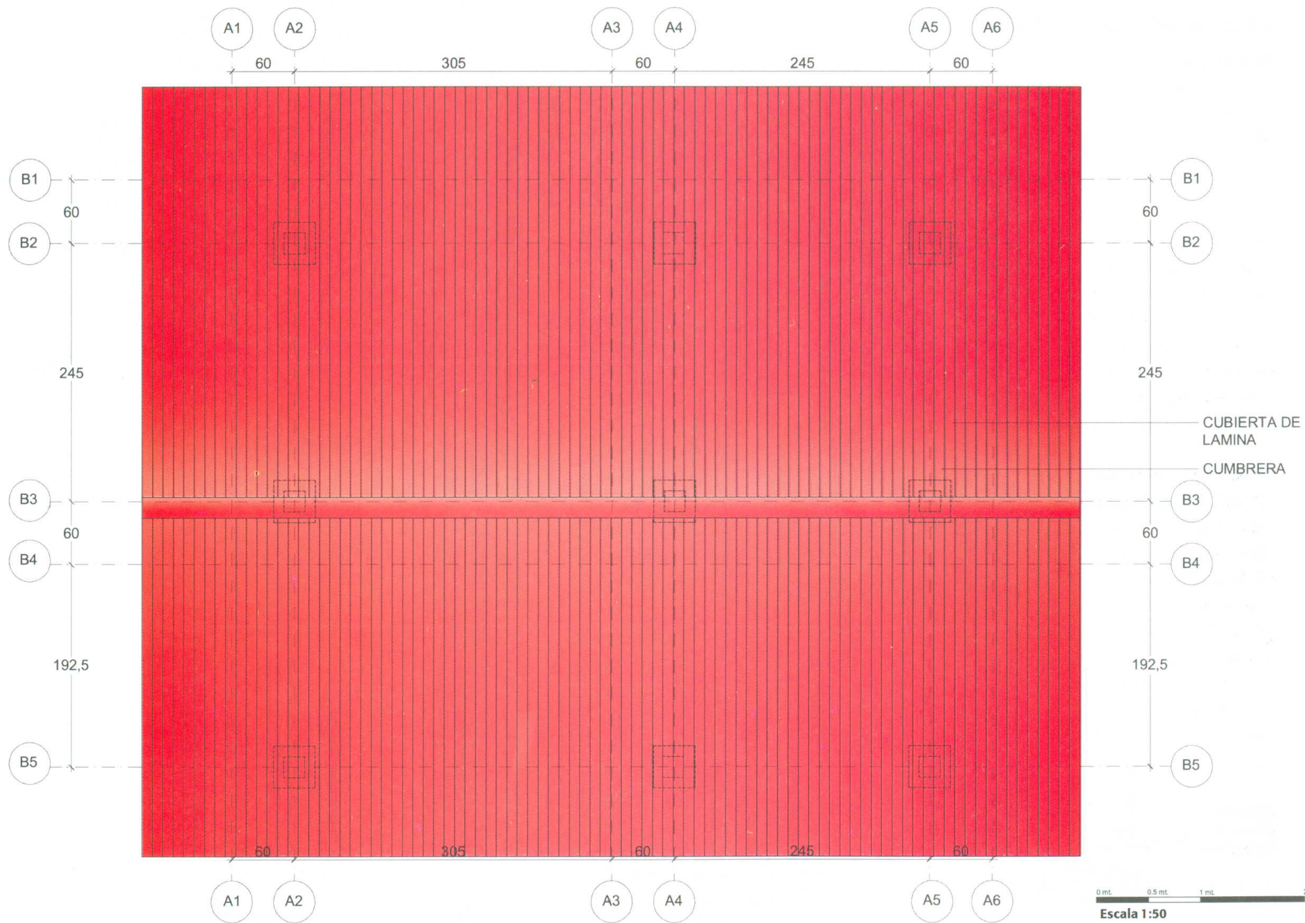
PLANTA ESTRUCTURAL TECHO (ARMAZÓN)
