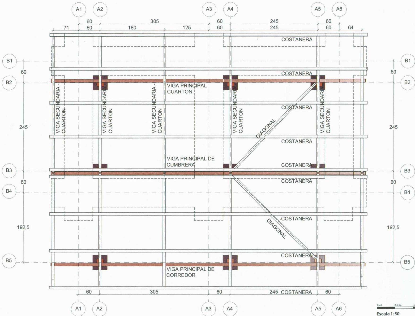
PLANTA ESTRUCTURAL TECHO (ARMAZÓN)
