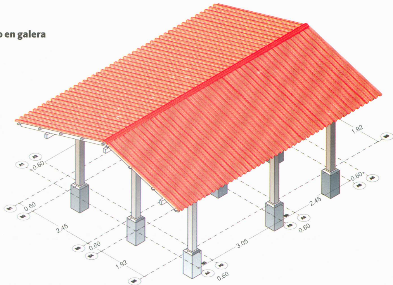
CUBIERTA DE TECHO – VISTA TRIDIMENSIONAL
