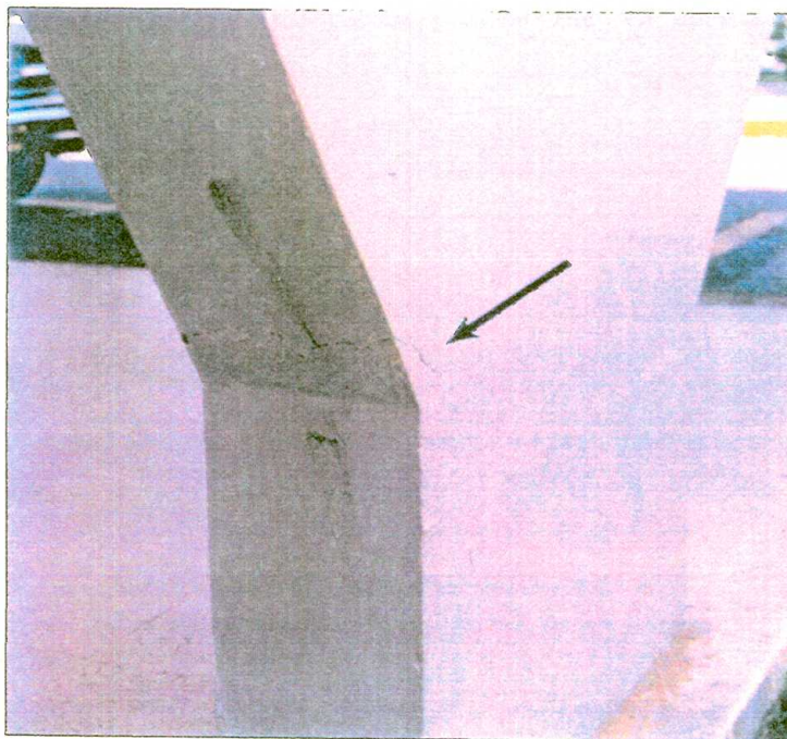
FOTO 14 Detalle de la Columna Fisurada (Foto 13)
