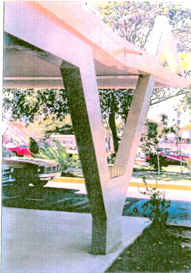
FOTO 13 Columna Fisurada de la pérgola en la entrada principal del Hospital (véase Foto 4).
