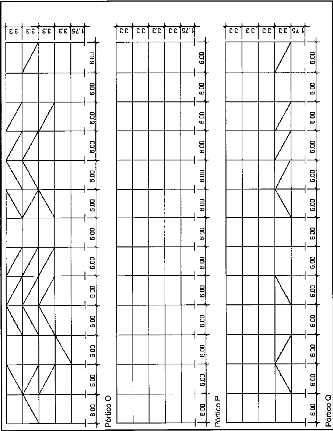
Figura 42. Pórticos longitudinales. Bloque de Hospitalizados 2. (Edificio 1).
