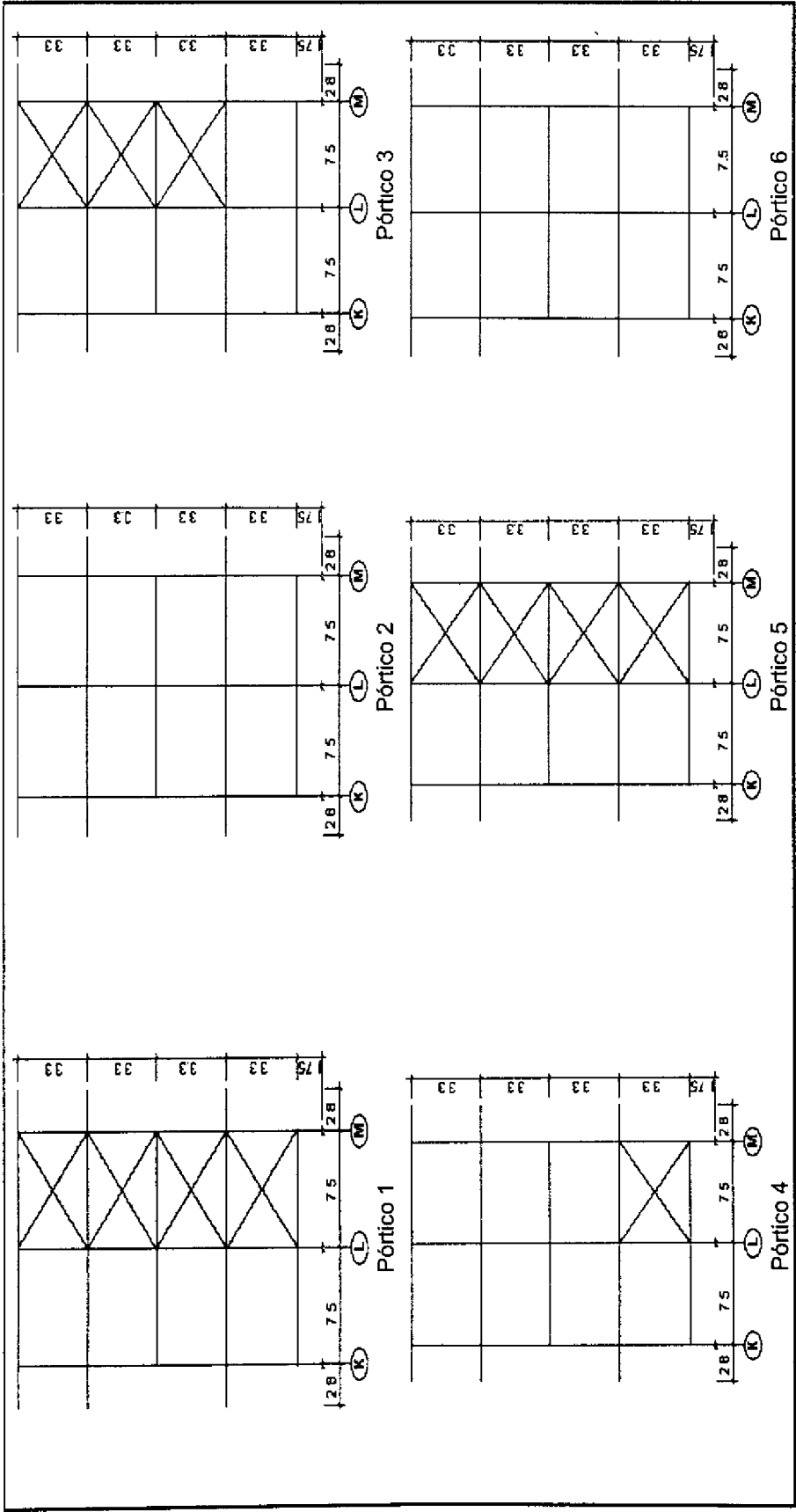
Figura 31. Pórticos transversales del 1 – 6. Bloque de Hospitalizados 1. (Edificio 1).
