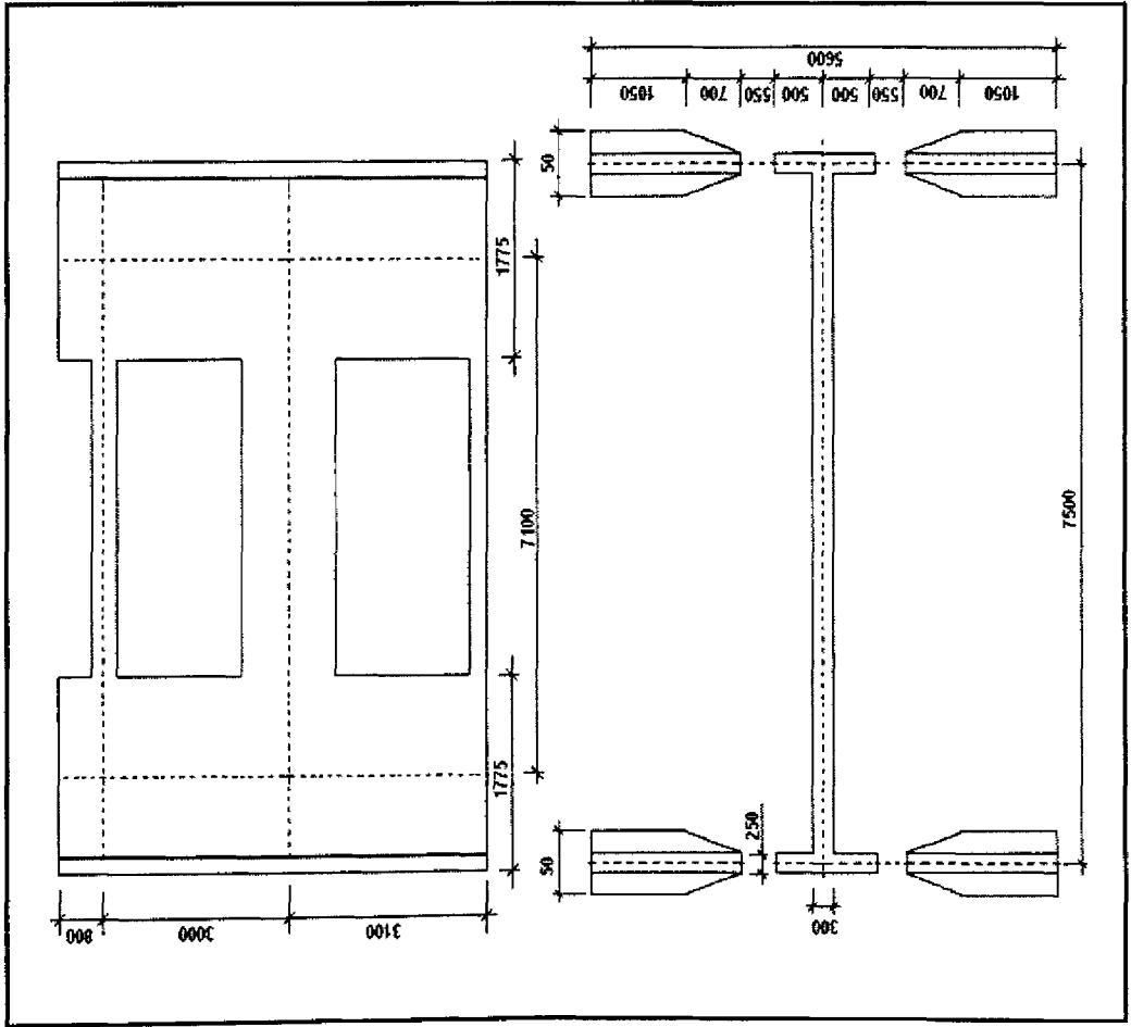
Figura 47. Detalles de los timpanos H.
