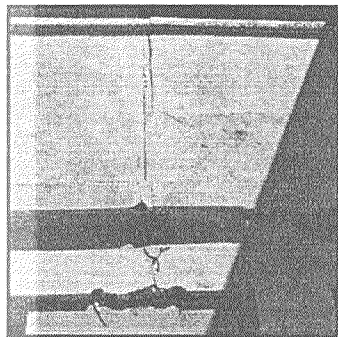
Foto 3. Grietas en paredes.
