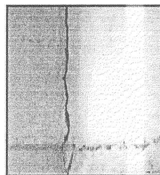
Foto 6. Grietas en paredes del local de lavandería.
