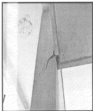
Foto 11. Grietas en paredes del local de lavandería.
