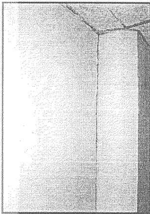
Foto 23. Asimetría en elevación, irregularidad en elevación del Bloque de Hospitalizados 1.
