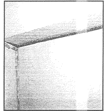
Foto 22. Grietas en paneles
