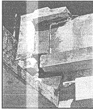
Foto 21. Grietas en uniones producto de asentamientos
