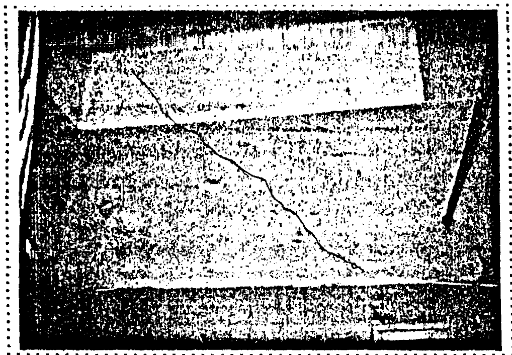
FOTO No. 9 : BLOQUE 'A'. Agrietamiento Tipo EA-1A. (V. Interna).
