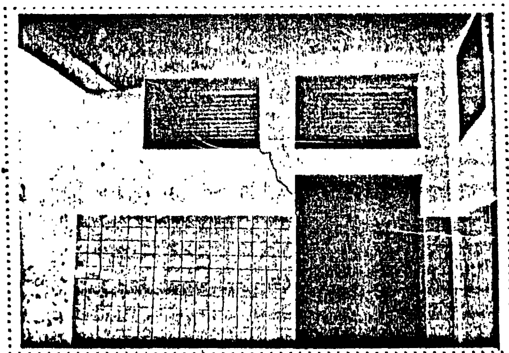
FOTO No. 11 : BLOQUE 'A'. Agrietamiento Tipo EA-2A.
