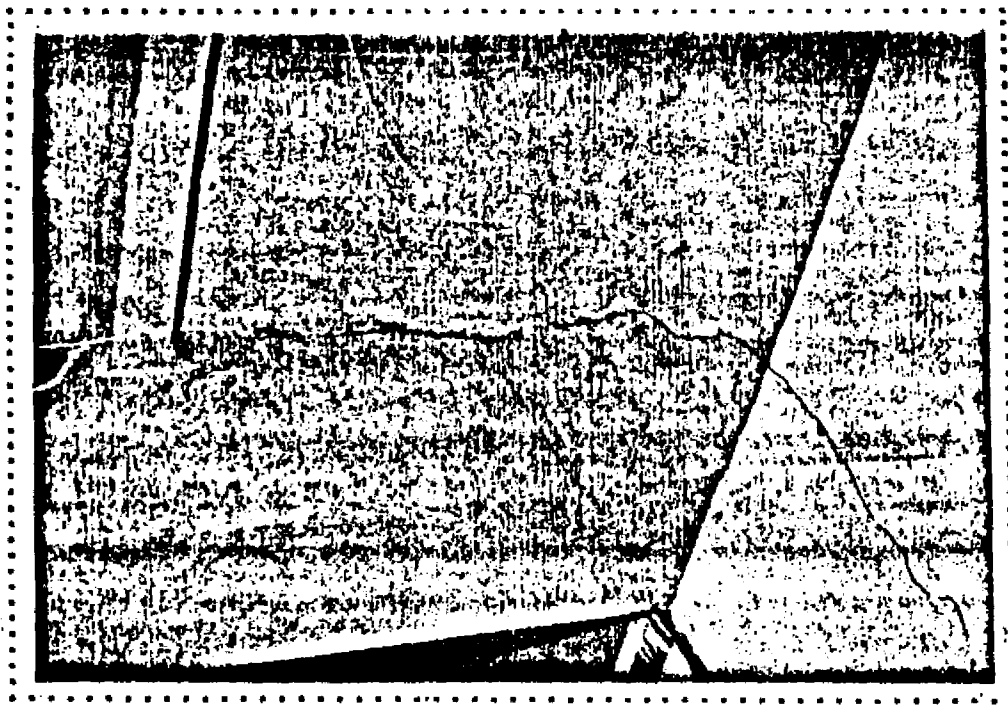
FOTO No. 28 : BLOQUE 'B'. Estado de Agrietamiento Tipo EA-5C.
