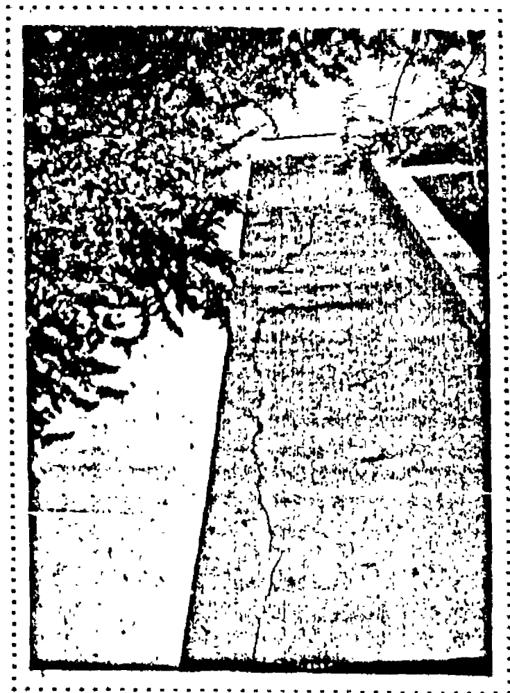
FOTO No. 56 : BLOQUE "c". Estado de Agrietamiento Tipo EA-6B.
