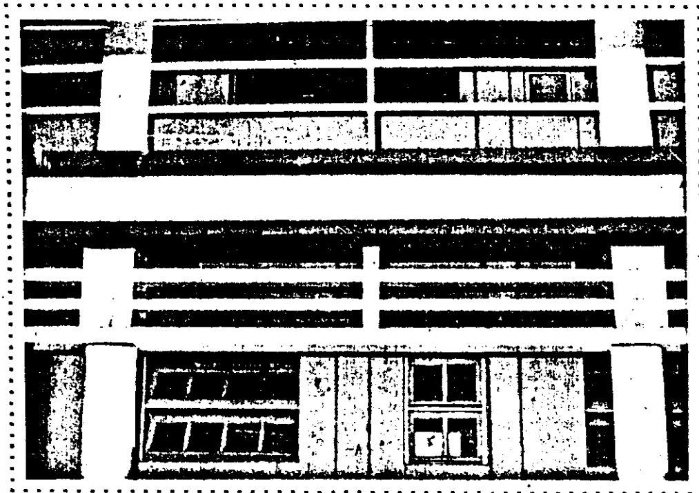
FOTO No. 43 : BLOQUE 'C'. Detalle Tipico Viga-Columna. Pasillo Central,
