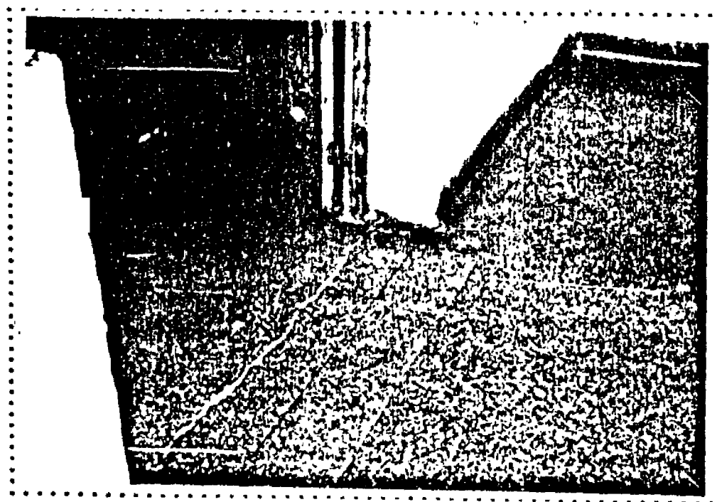
FOTO No. 37 : Pasarela B-C. Estado de Agrietamiento Tipo EA-3A.
