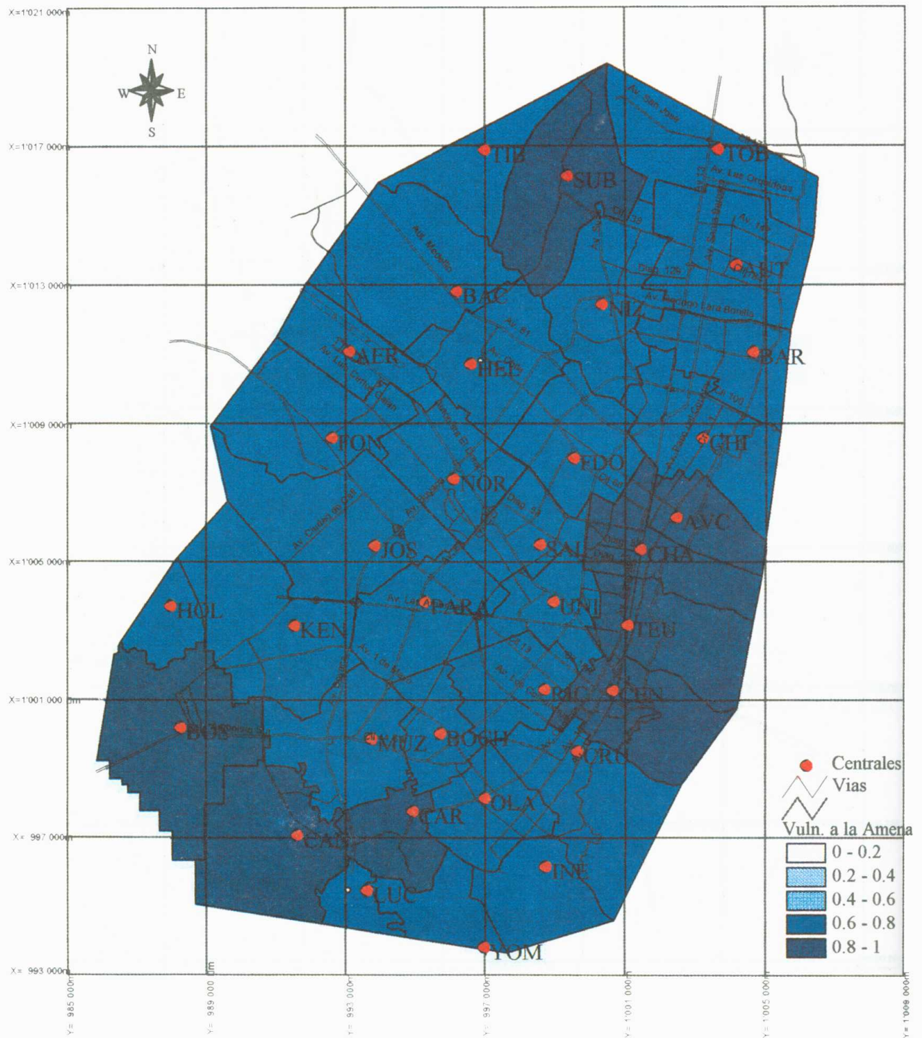
FIGURA 4.14 VULNERABILIDAD DE CENTRALES TELEFÓNICAS A LA AMENAZA SISMO CERCANO MODERADO (0.12g).
