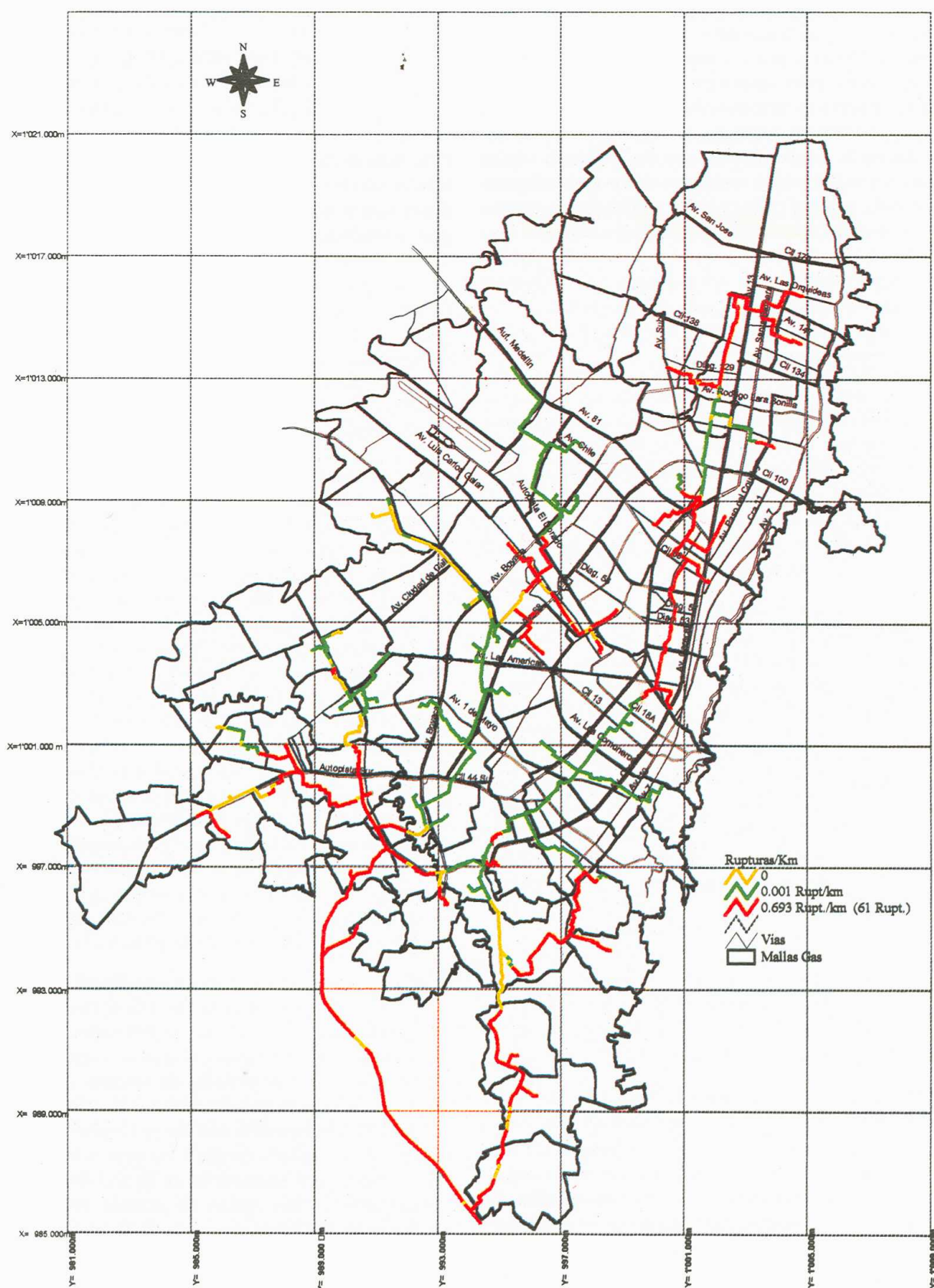
FIGURA 4.17 DAÑOS ESPERADOS EN LA RED DE GAS PARA EL SISMO CERCANO FUERTE (0.2g)
