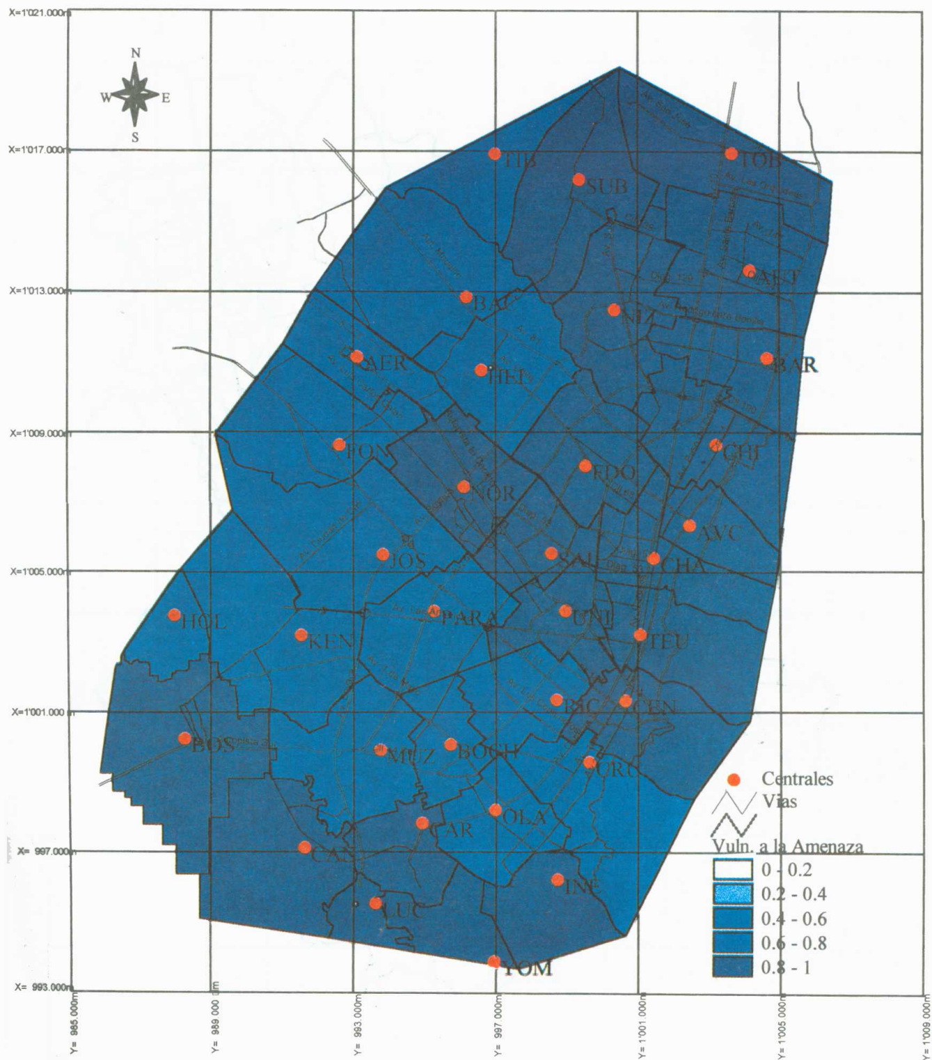
FIGURA 4.15 VULNERABILIDAD DE CENTRALES TELEFÓNICAS A LA AMENAZA SISMO CERCANO FUERTE (0.2g).
