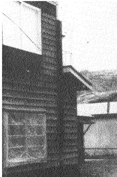
Fotografía 5. Refuerzo de columna de gran altura con adición de columna.
