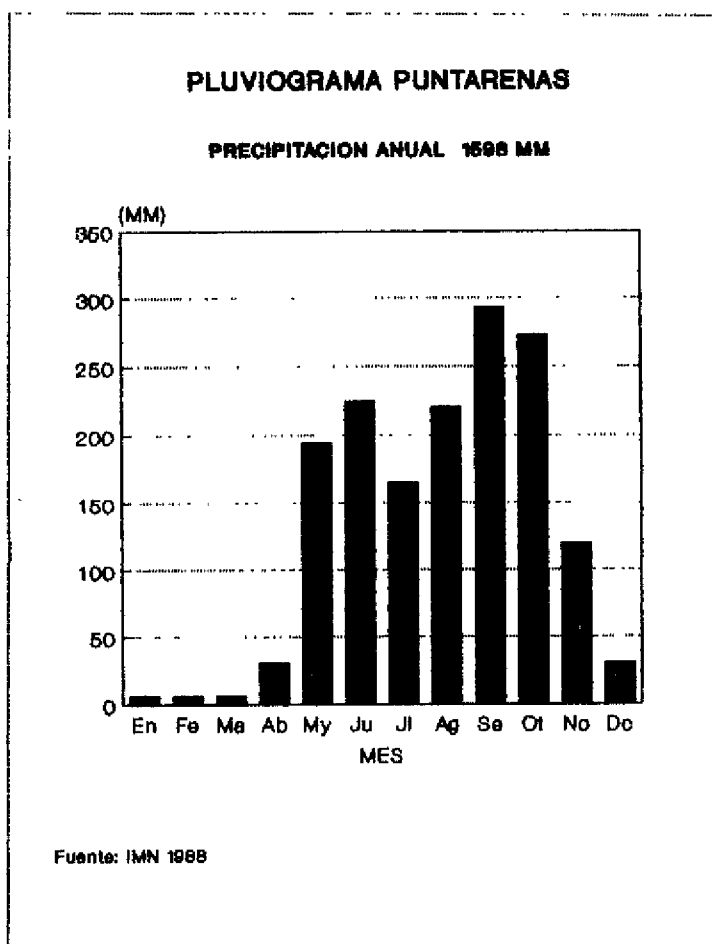
Fig. 4: Pluviograma Puntarenas
