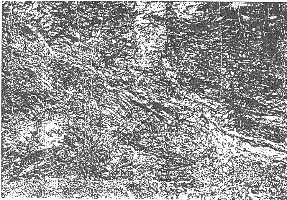
23. Afloramiento de Limolitas Terciarias En la margen derecha del Río Navarro con falla con desplazamiento de 50 cm.
