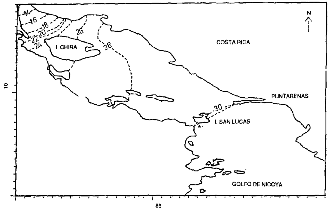
FIGURA 2. Salinidad (%) en superficie. Estación seca - Marea baja.
