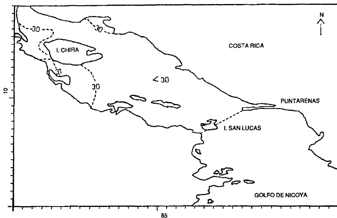
FIGURA 6. Temperatura (°C) en superficie. Estación seca – Marea baja.
