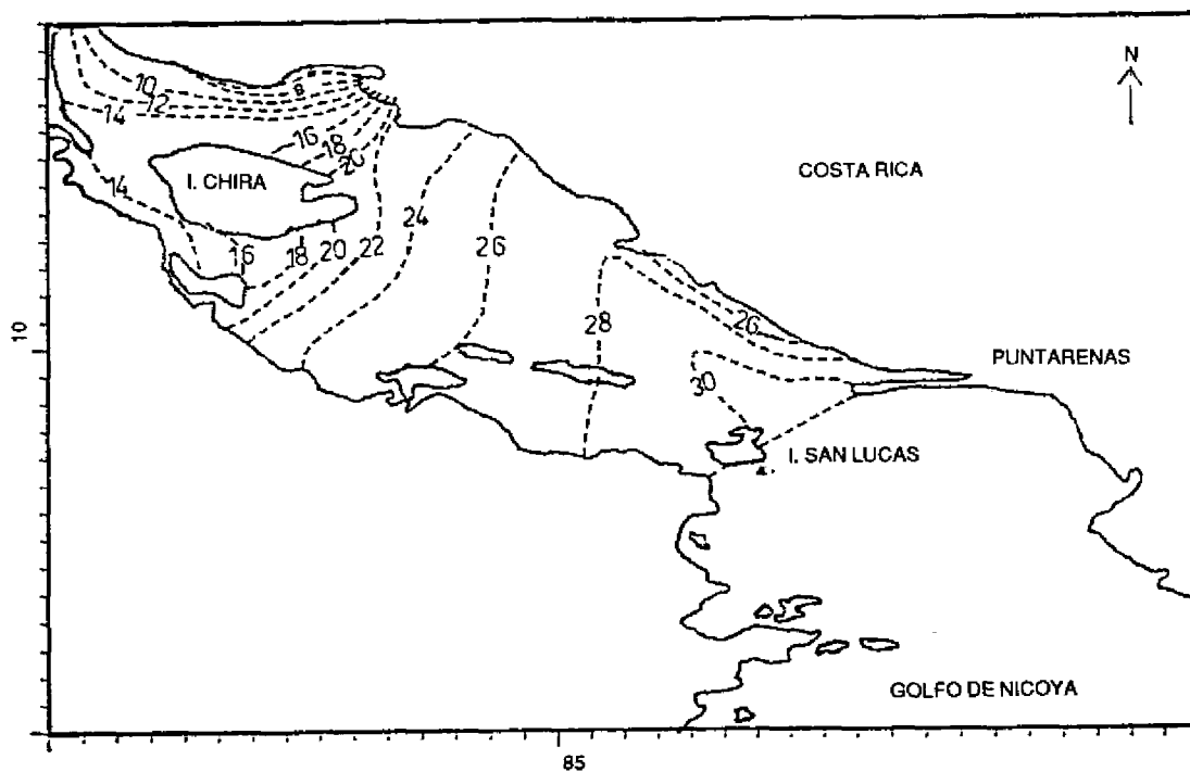
FIGURA 11. Salinidad (%) en el fondo. Estación lluviosa – Marea baja.
