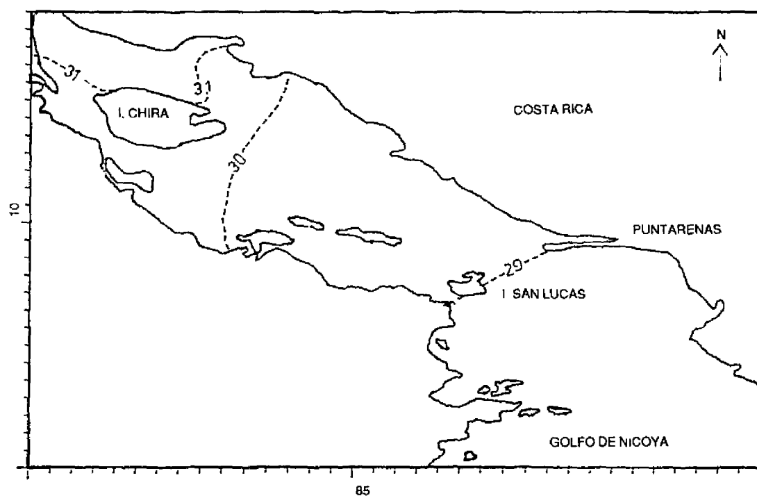
FIGURA 8. Temperatura (°C) en superficie. Estación seca – Marea alta.
