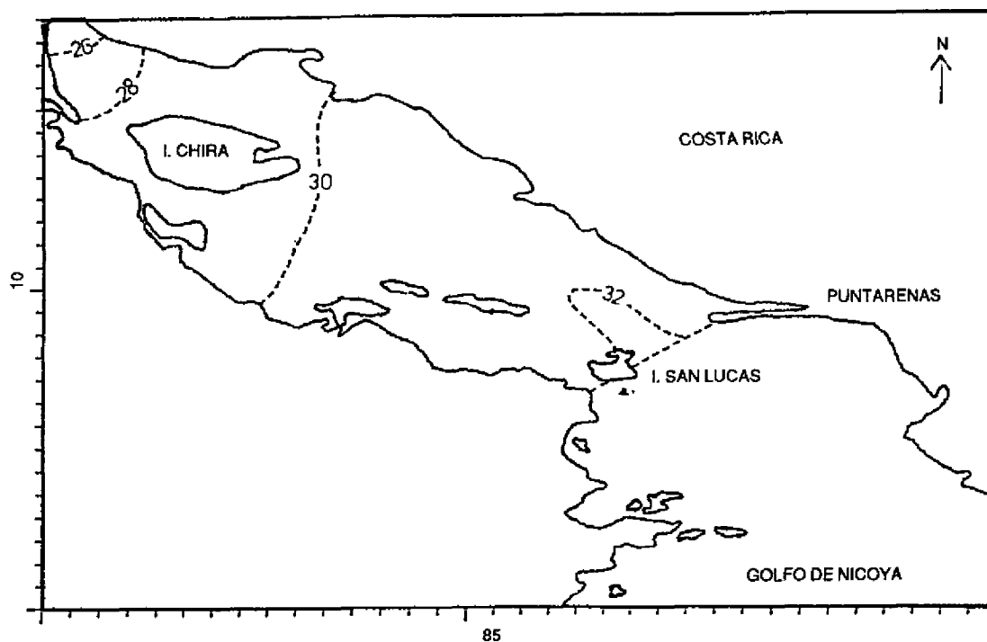
FIGURA 13. Salinidad (%) en el fondo. Estación lluviosa – Marea alta.
