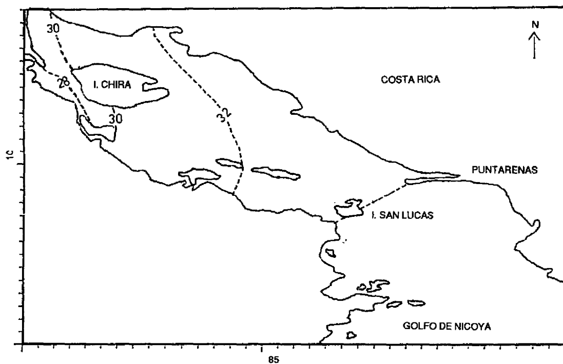
FIGURA 5. Salinidad (%) en al fondo – Esta- ción seca – Marea alta.
