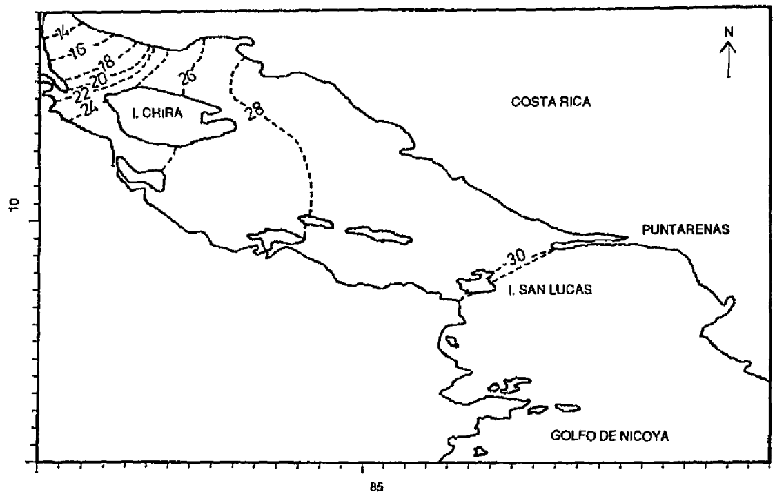
FIGURA 3. Salinidad (%) en el fondo. Estación seca - Marea baja.
