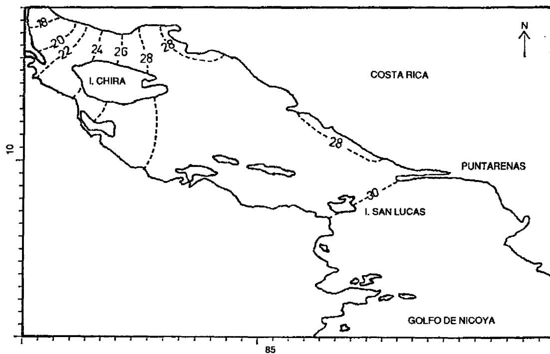
FIGURA 12. Salinidad (%) en superficie. Estación lluviosa – Marea alta.
