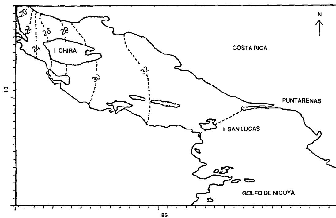
FIGURA 4. Salinidad (%) en superficie – Estación seca – Marea alta.
