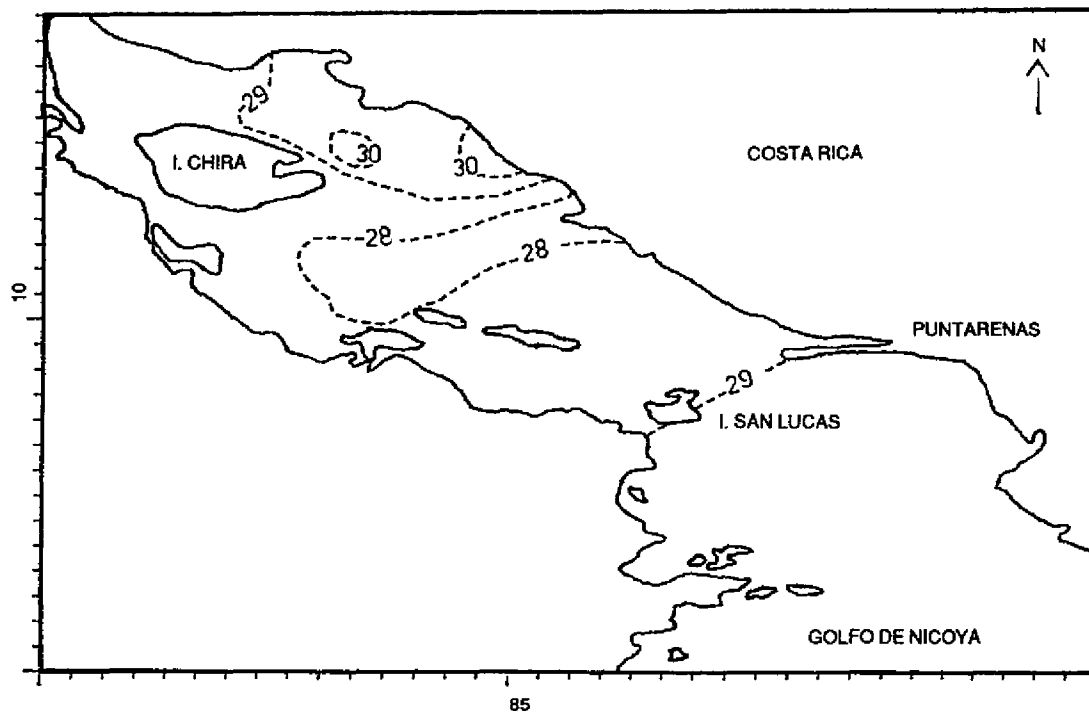
FIGURA 14. Temperatura (°C) Superficie. Estación lluviosa – Marea baja.
