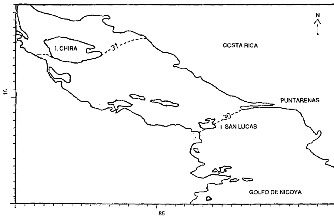
FIGURA 16 Temperatura (°C) en Superficie Estación lluviosa - Marea alta.
