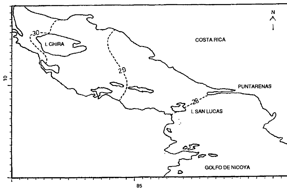
FIGURA 9. Temperatura (°C) en el fondo. Estación seca – Marea alta.
