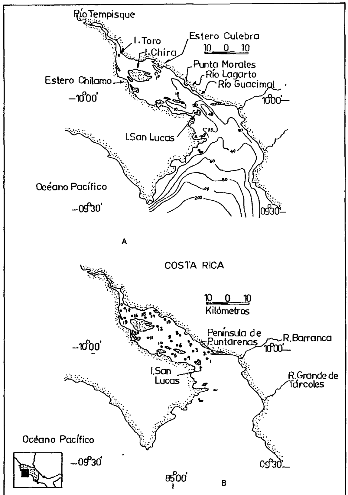
FIGURA 1. Golfo de Nicoya; A, características geográficas y estratigráficas; B, ubicación de las estaciones de estudio.
