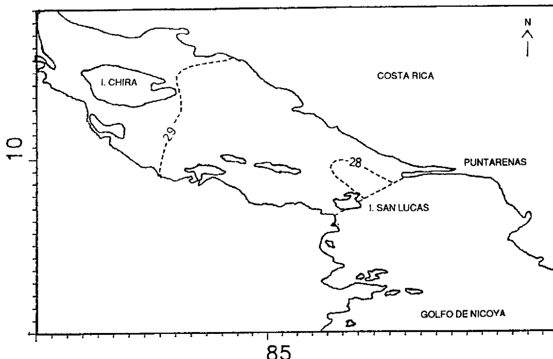
FIGURA 17. Temperatura (°C) en el fondo. Estación lluviosa – Marea alta.
