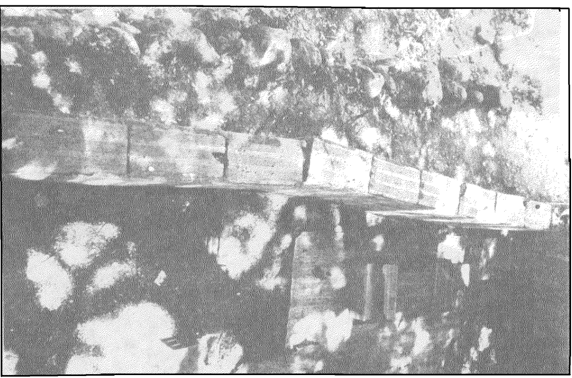
Fig. 10. Desplazamiento dextral de la pared de una vivienda de Muelle de Cariaco.
