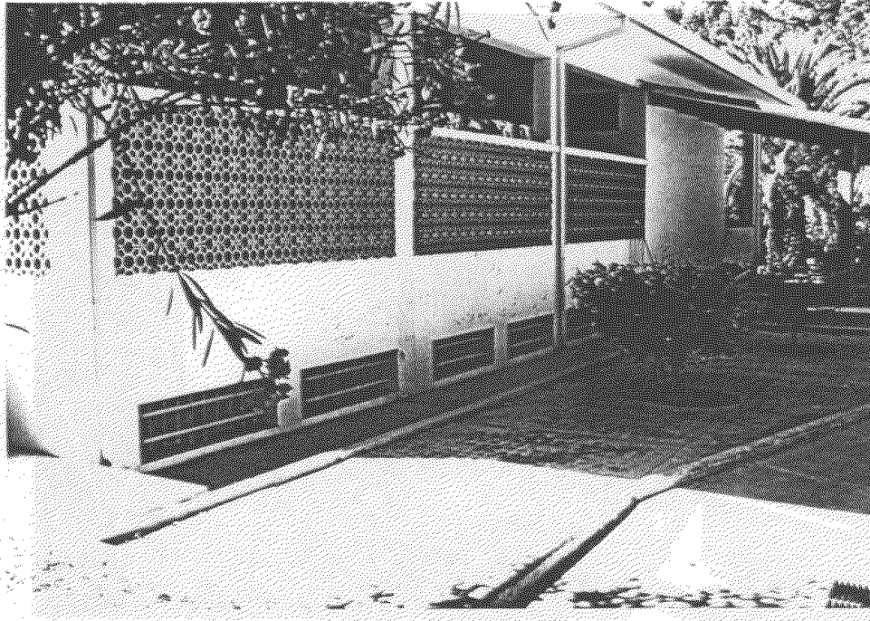
Foto 7. Vista de la fachada longitudinal posterior del Hospital Bertol de Aiquile
