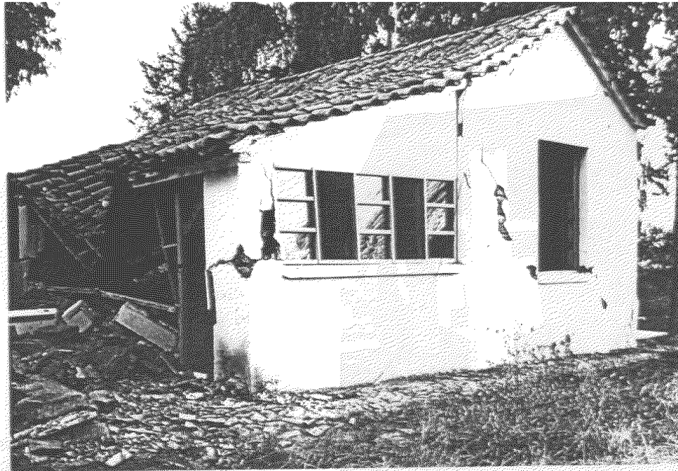
Foto 21. Daños edificio de cocina y lavandería Hospital Carmen López
