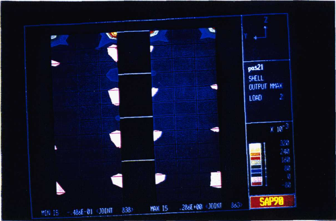
MOMENTOS EN PANELES DE PORTICO PERPENDICULAR A FACHADAS
