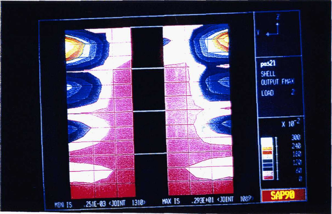
CORTANTES EN PANELES DE PORTICO PERPENDICULAR A FACHADAS
