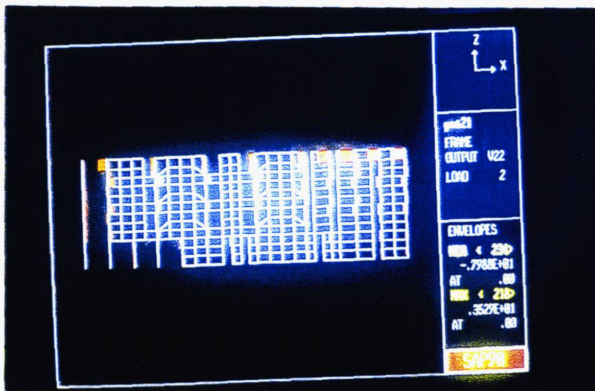
ESFUERZOS EN COLUMNAS DE PORTICO INTERIOR PROPUESTO
