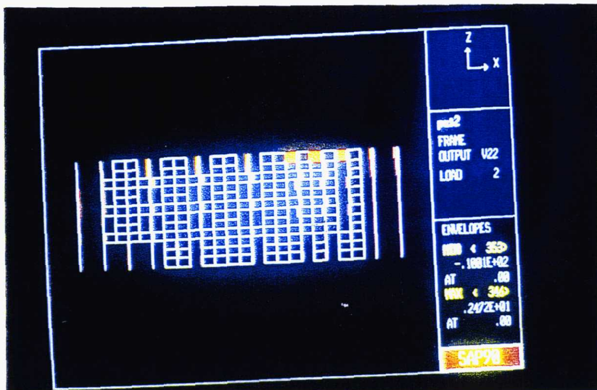
ESFUERZOS EN COLUMNAS DE PORTICO INTERIOR EXISTENTE
