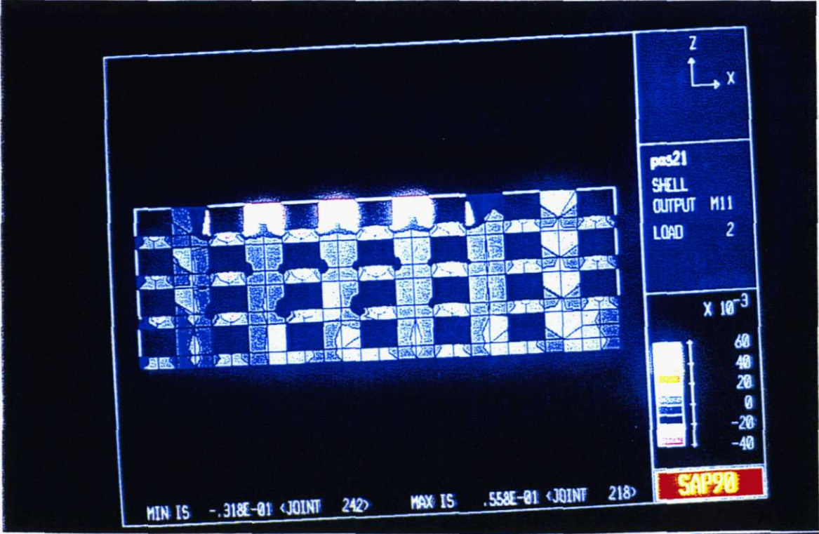
MOMENTOS EN PORTICOS INTERIORES EN ESTRUCTURA EXISTENTE
