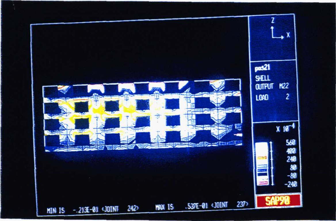
MOMENTOS EN PORTICOS INTERIORES EN ESTRUCTURA PROPUESTA
