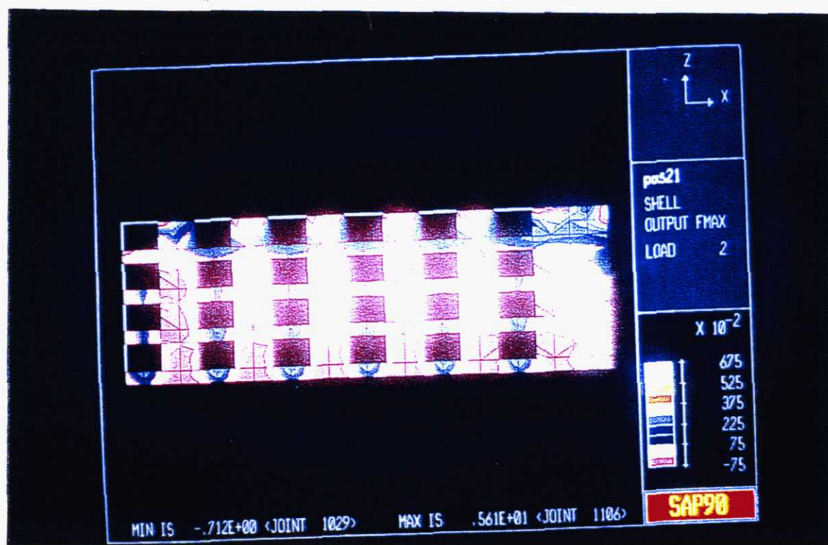
ESFUERZOS CORTANTES EN PANELES DE FACHADA PROPUESTA
