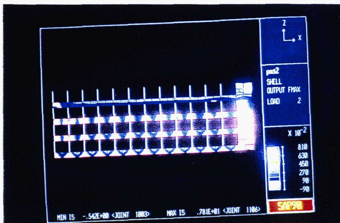
ESFUERZOS CORTANTES EN PANELES DE FACHADA EXISTENTE
