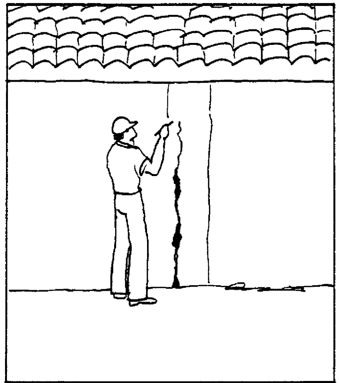
Marque el área para ser reparada
