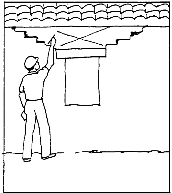
Marque el área sobre las grietas y el dintel
