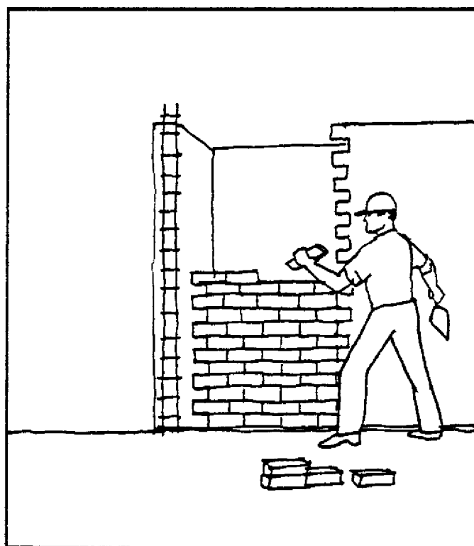
Coloque castillo (armazón), reconstruya la pared, arme formaleta y funda columneta
