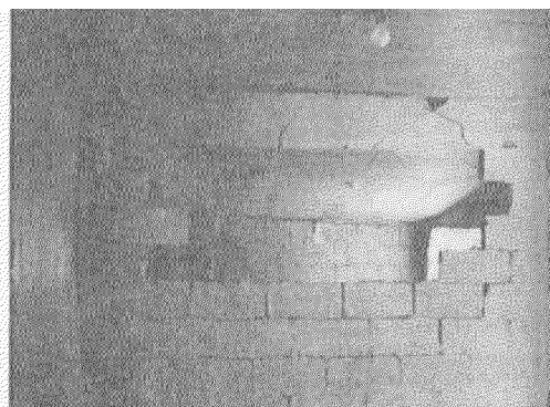
Figura N° 10 Pared sin acero de refuerzo ni viga corona.
