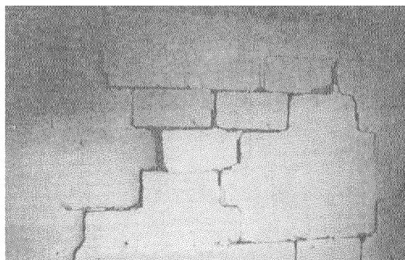
Figura N° 9 Bloques fuera del plano de la pared.
