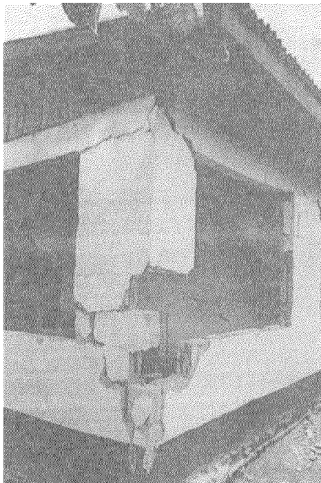
Figura N° 7 Falla en unión de paredes.
