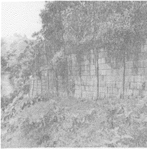
Figura Nº 19 Muro de retención deformado.
