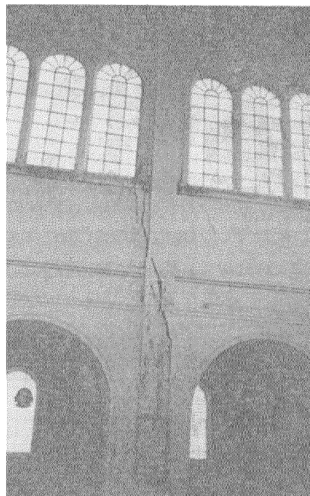
Figura Nº 22 Daños en la Iglesia de Puriscal.
