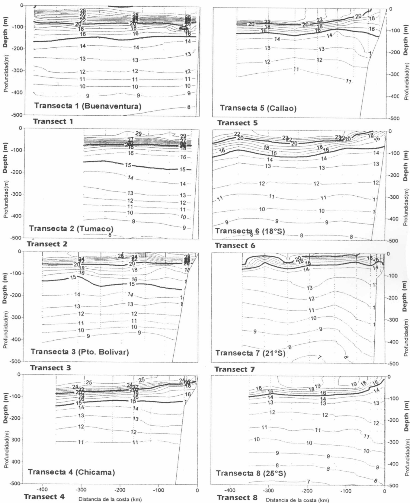
Figura 9.- Distribución vertical de la temperatura (°C). Transectas perpendiculares a la costa. Mayo 1998.
