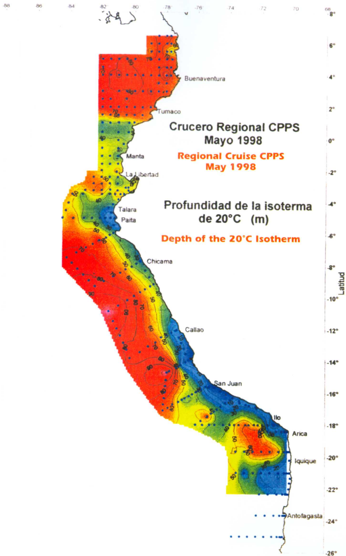
Figura 7.- Profundidad de la Isotherma de 20°C. Mayo 1998. Crucero Regional CPPS Chart 7.- Depth of the 20°C isotherm. May 1998. Regional Cruise CPPS
