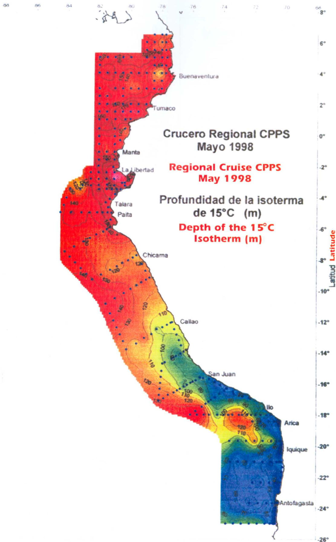
Figura 8.- Profundidad de la isoterma de 15°C. Mayo 1998. Crucero Regional CPPS Chart 8.- Depth of the 15°C isotherm. May 1998. Regional Cruise 1998
