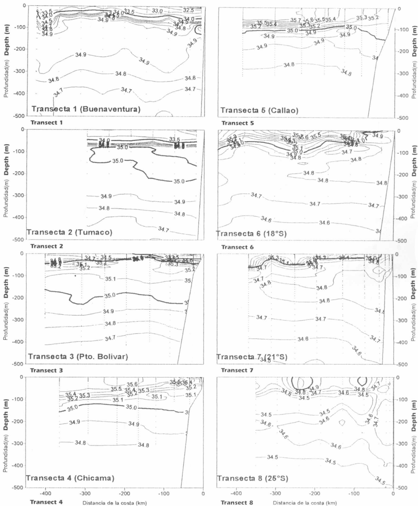
Figura 10.- Distribución vertical de salinidad (ups). Transectas perpendiculares a la costa. Mayo 1998 Chart 10.- Vertical distribution of salinity .Transects perpendicular to the coast.May 1998
