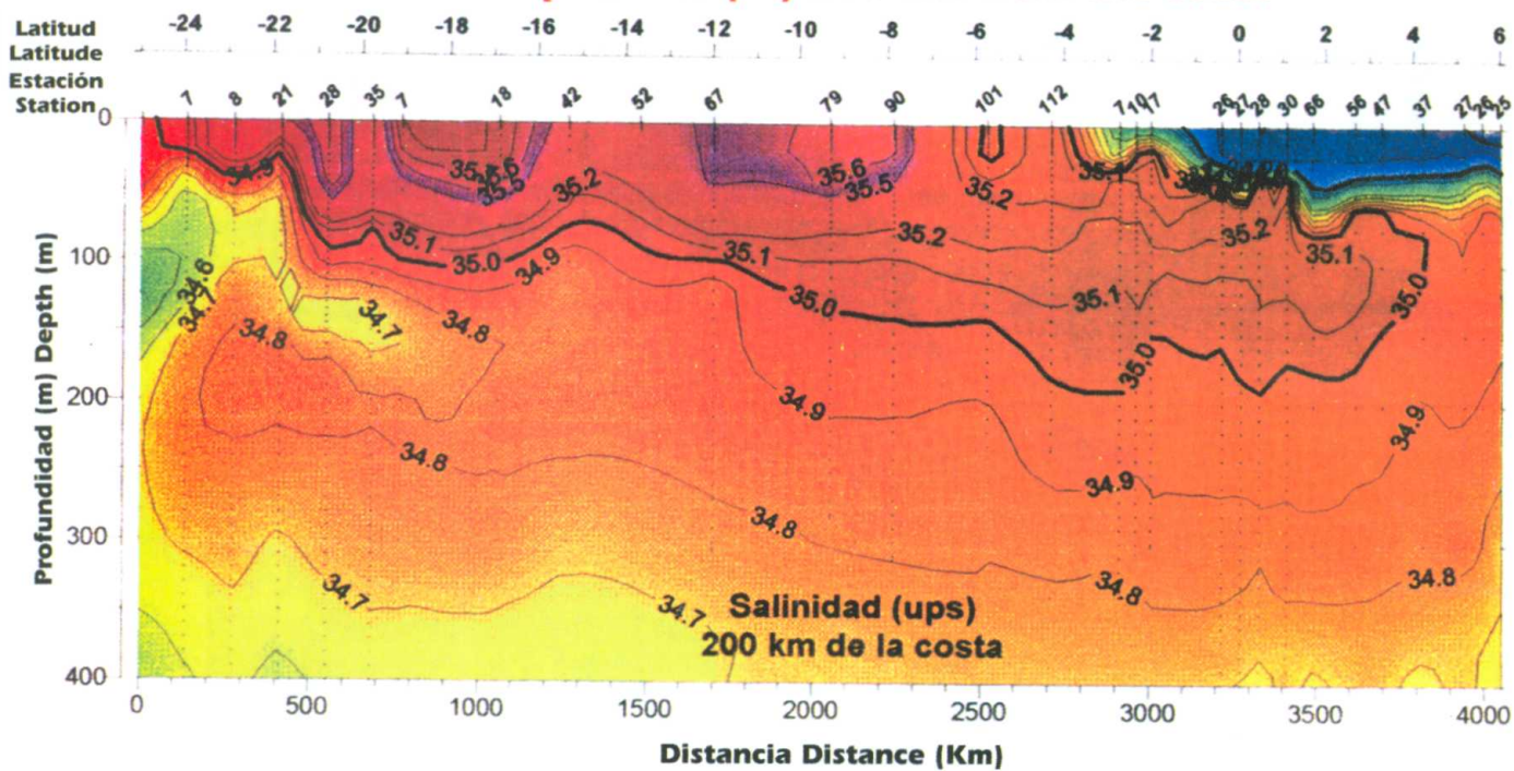
Figura 11.- Distribución vertical de temperatura y salinidad a 200 km a lo largo de la costa de sudamérica. Mayo 1998
