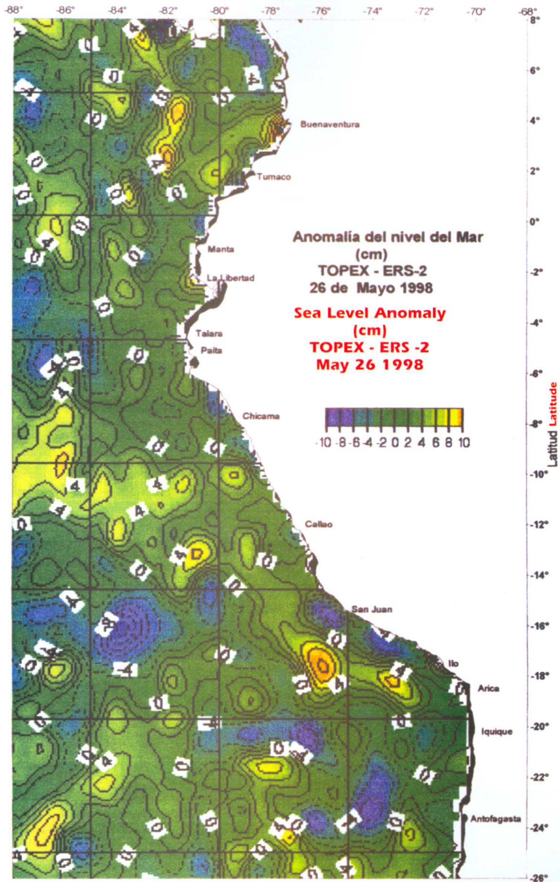
Figura 12.- Anomalía del nivel del mar (cm). Satélites TOPEX y ERS-2. Análisis del CCAR
