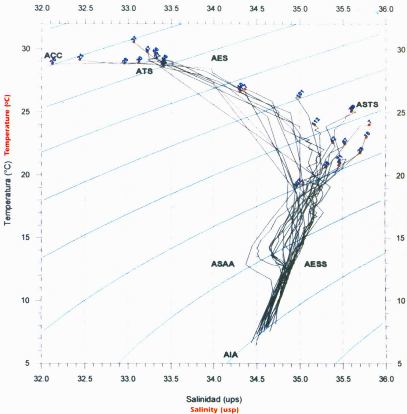
Figura 13.- Diagrama t-s de las estaciones en transecta paralela a la costa a 200 km. Mayo 1998 Chart 13.- T-S Diagram of the stations on the 200 km transect parallel to the Coast. May 1998
