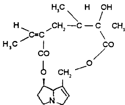
Senecionina C_{18}H_{25}NO_5 No.de registro del CAS: 130-01-8
