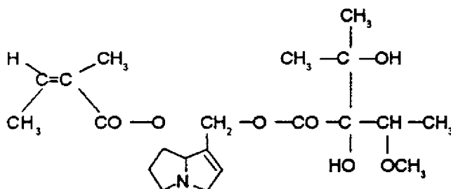
Retrorsina C_{18}H_{25}NO_3 No.de registro del CAS:480-54-6
