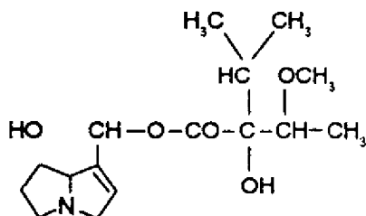
Monocrotalina C_{16}H_{23}NO_6 No.de registro del CAS: 315-22-0
