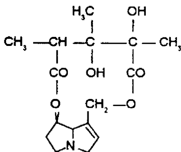
Senecionina C_{18}H_{25}NO_5 No.de registro del CAS: 130-01-8
