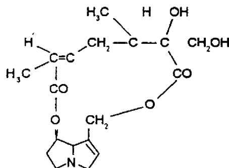
Retrorsina C_{18}H_{25}NO_3 No.de registro del CAS:480-54-6
