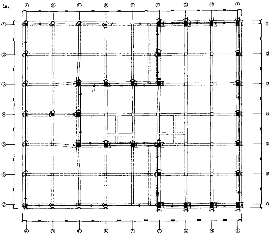
PLANTA LOSA PRIMER PISO ALTO BLOQUE PRINCIPAL - BLOQUE # 1
