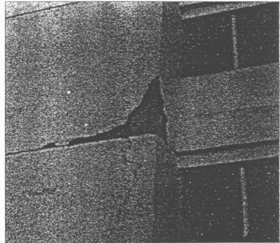
AREA DE GINECOLOGÍA, DESPLOME DE MAMPOSTERÍA NO ARRIOSTRADA
