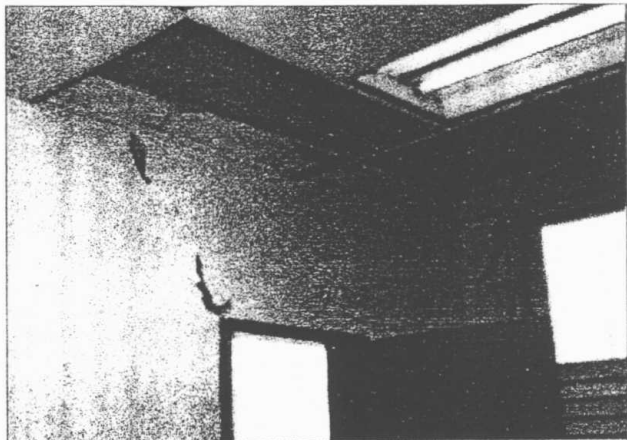
FALLA DE CORTE EN ESQUINA POR AUSENCIA DE DINTEL SOBRE LA PUERTA
