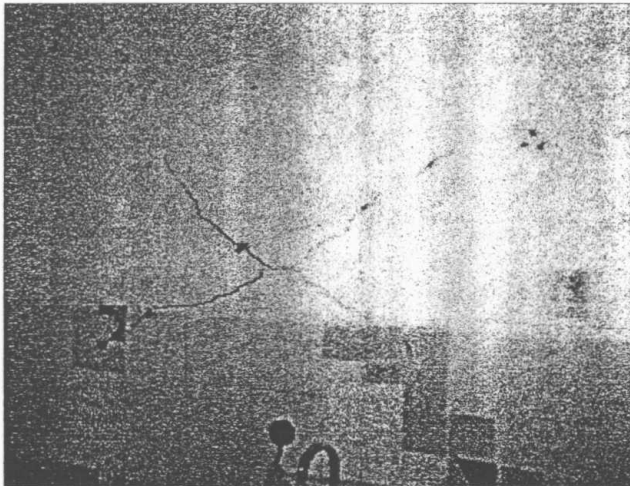
AREA DE NEONATOLOGÍA, PRIMER PISO FALLA DE CORTE EN CRUZ EN LA MAMPOSTERÍA
