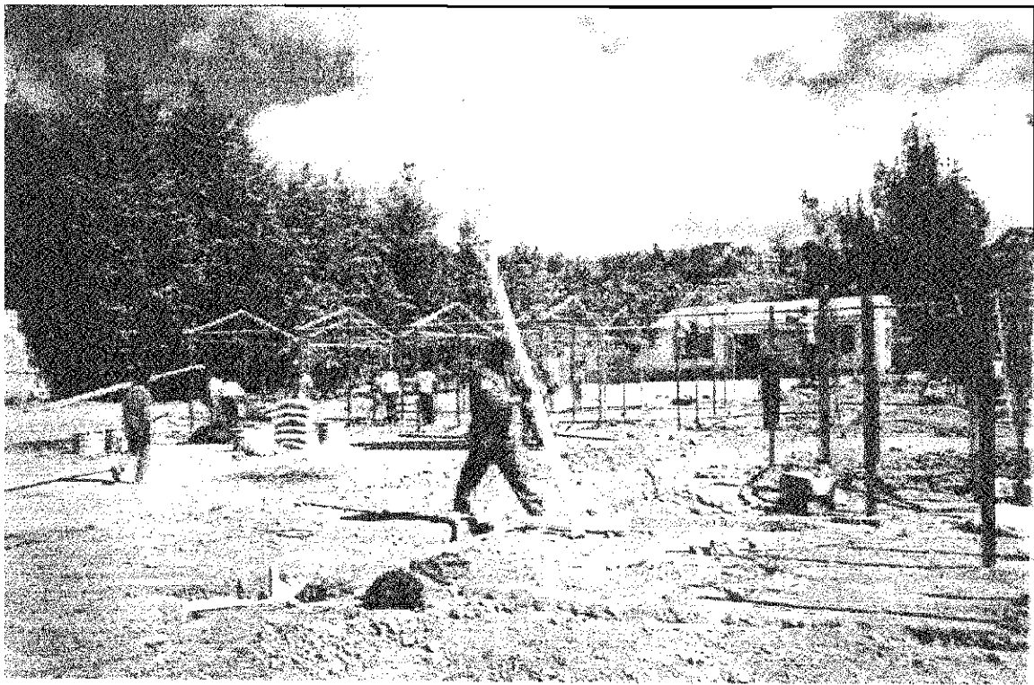
9.- Instalación de Drenajes a la red de alcantarillado.
