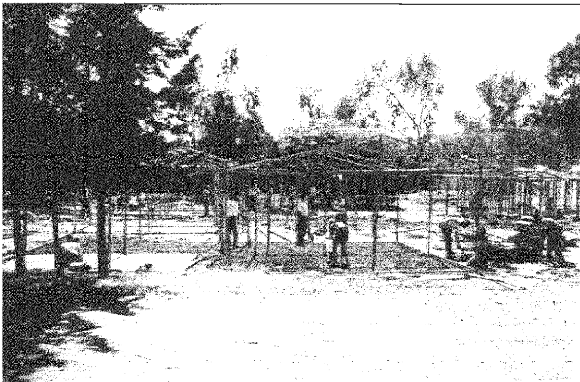
13.- Preparación de pisos de cemento.
