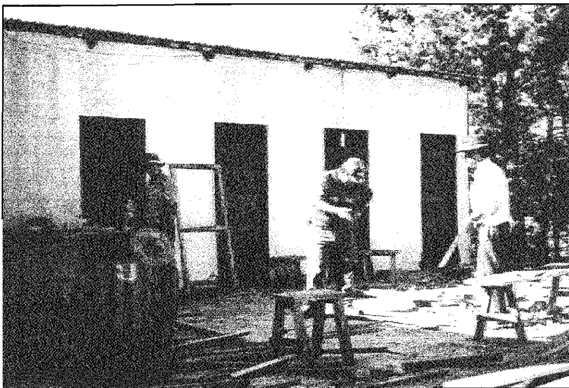
12.- Dirección Técnica para el armado de Estructuras de Madera.
