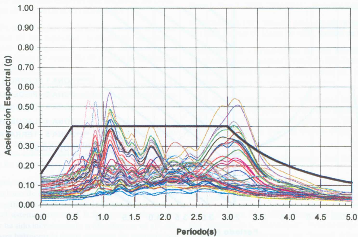
FIGURA 3.24 ESPECTROS DE RESPUESTA Y DE DISEÑO ZONA 4 - LACUSTRE B
