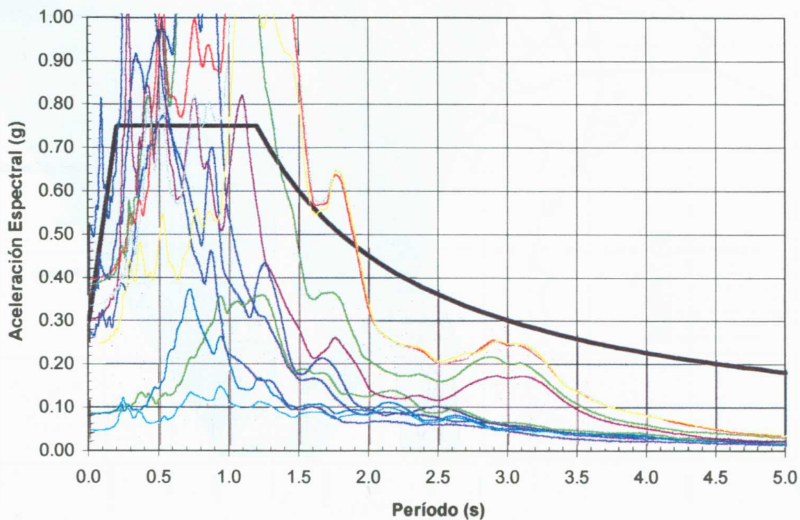
FIGURA 3.22 ESPECTROS DE RESPUESTA Y DE DISEÑO ZONA 2 - PIEDEMONTE
