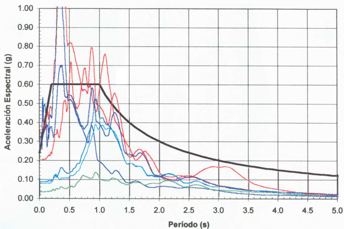
FIGURA 3.21 ESPECTROS DE RESPUESTA Y DE DISEÑO ZONA 1-CERROS
