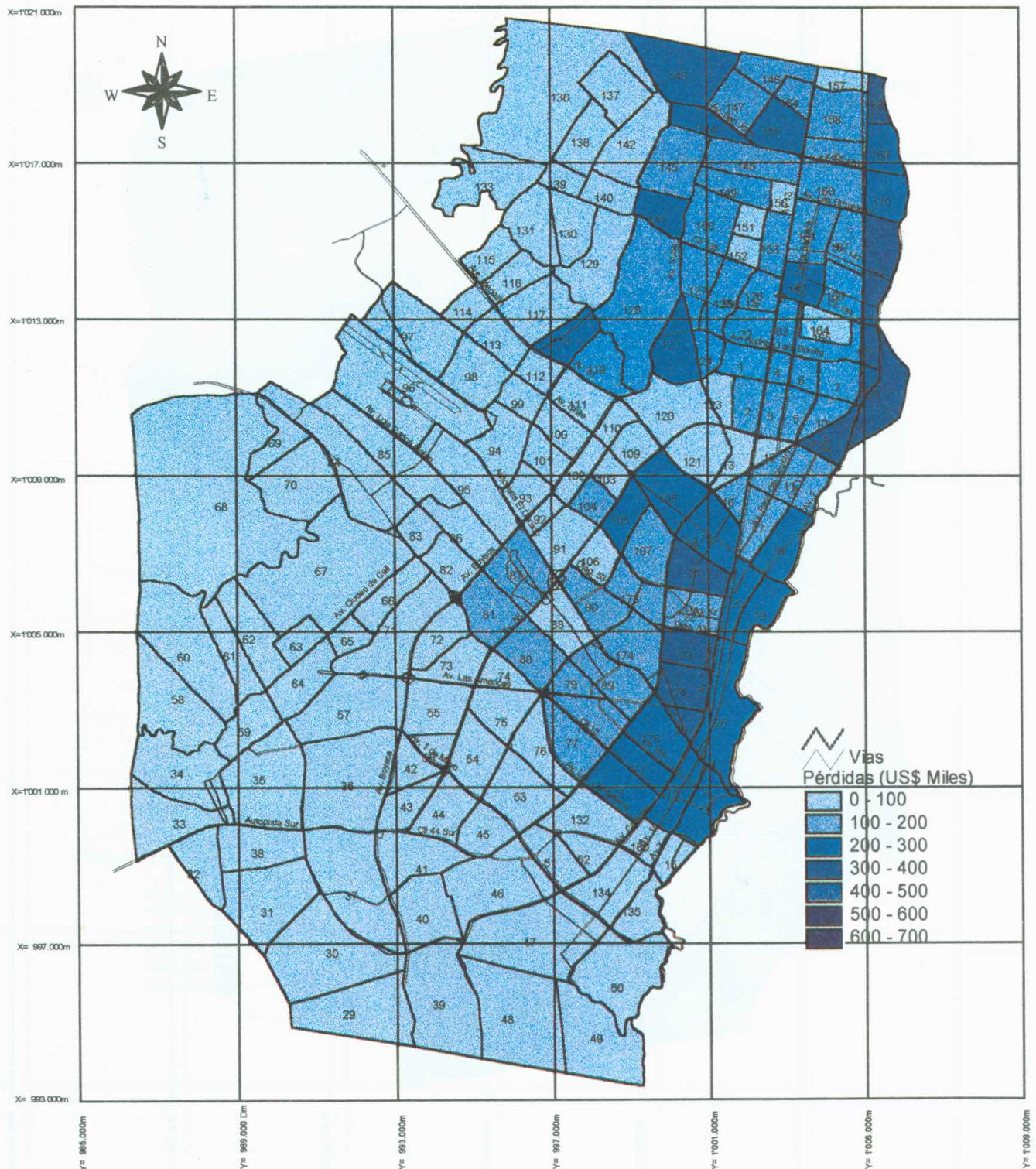
FIGURA 4.5 PÉRDIDAS ECONÓMICAS POR MANZANA SISMO CERCANO MODERADO (0.12g)
