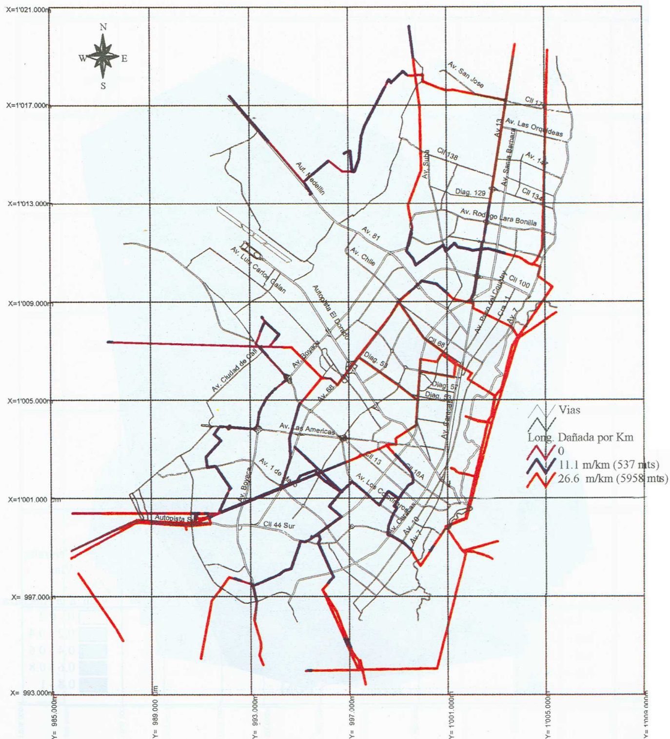
FIGURA 4.13 DAÑOS ESPERADOS EN LA RED DE ALTA TENSIÓN PARA EL SISMO CERCANO FUERTE (0.2g).
