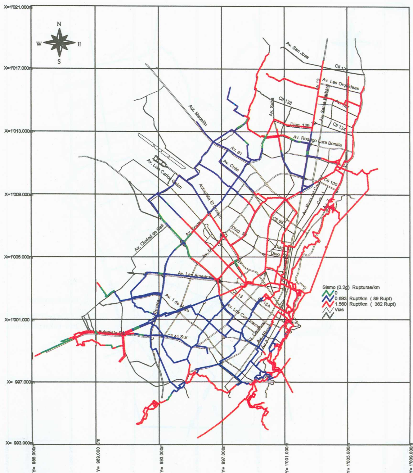
FIGURA 4.11 DAÑOS ESPERADOS EN LA RED DE ACUEDUCTO DEBIDOS AL SISMO CERCANO FUERTE (0.20g).
