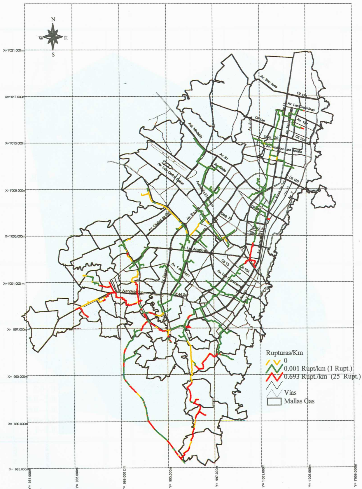
FIGURA 4.16 DAÑOS ESPERADOS EN LA RED DE GAS PARA EL SISMO CERCANO MODERADO (0.12g)
