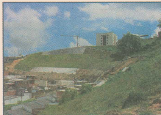
BARRIO EL TUCÁN. TRATAMIENTO DE ESTABILIDAD EN EJECUCIÓN.
