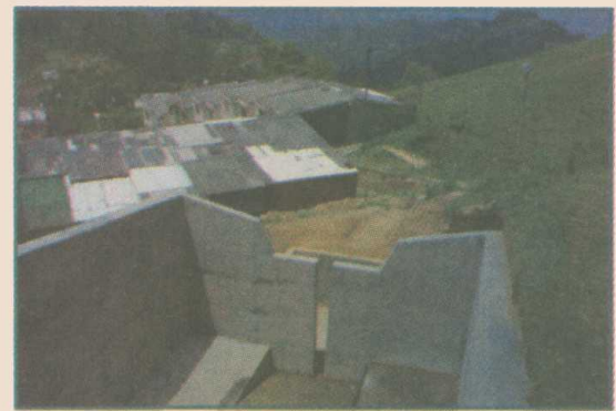
BARRIO MONTANA. (FOTOGRAFÍA TOMADA DESPUÉS DE CONSTRUIR LA OBRA DE ESTABILIDAD).
