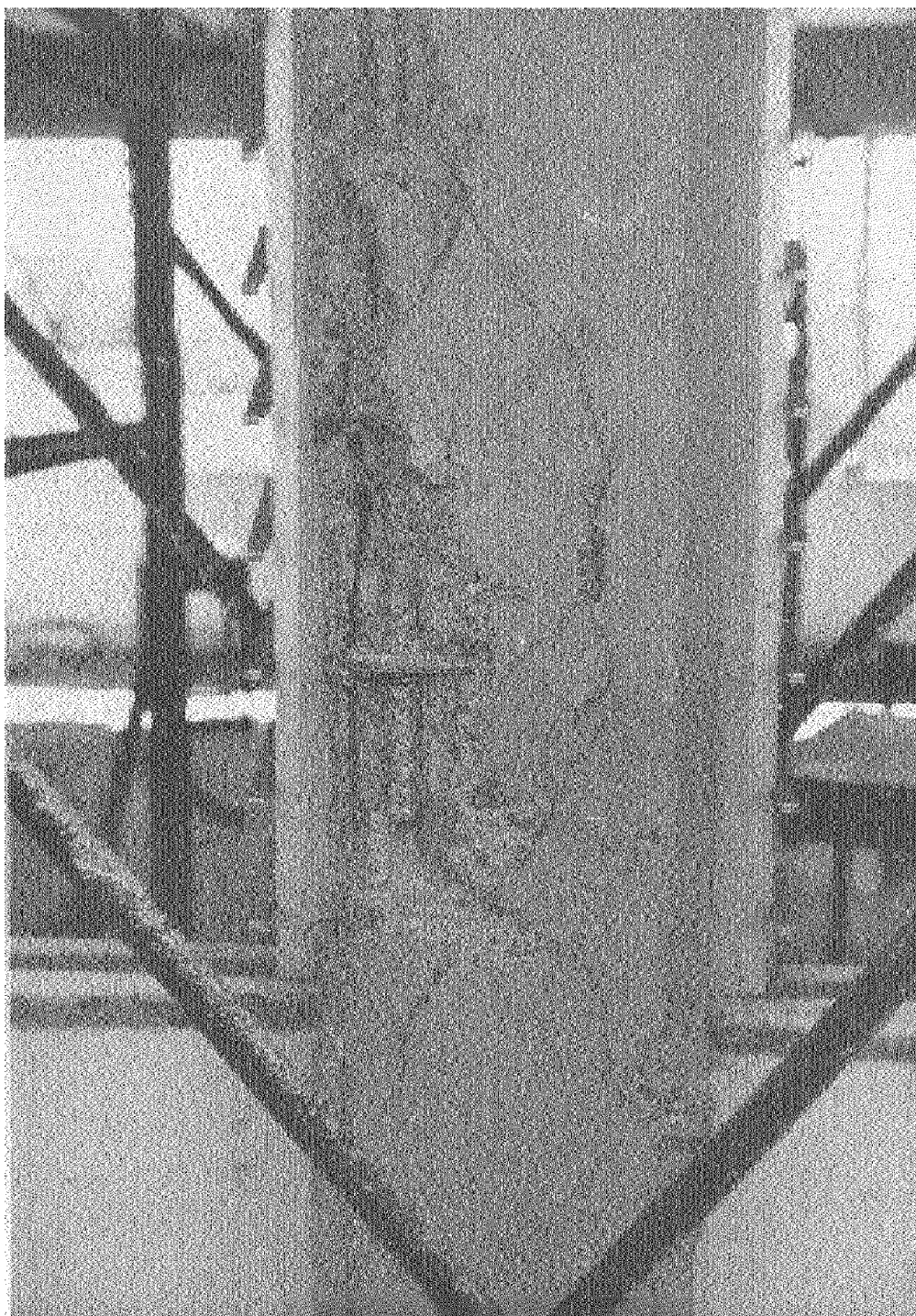
Foto 2.- Columna localizada en la parte Norte de la edificación, mostrando falla por cortante [1].
