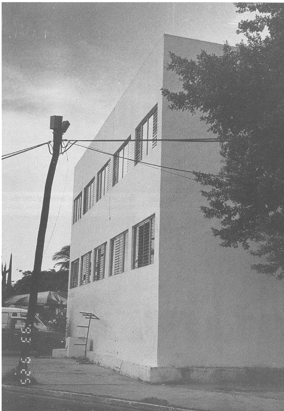
Foto 14.- Estructura de mampostería ubicada en la parte Este del complejo, en donde se observa el refuerzo de castillos (columnas) y la reparación de los muros de mampostería (septiembre de 1993).
