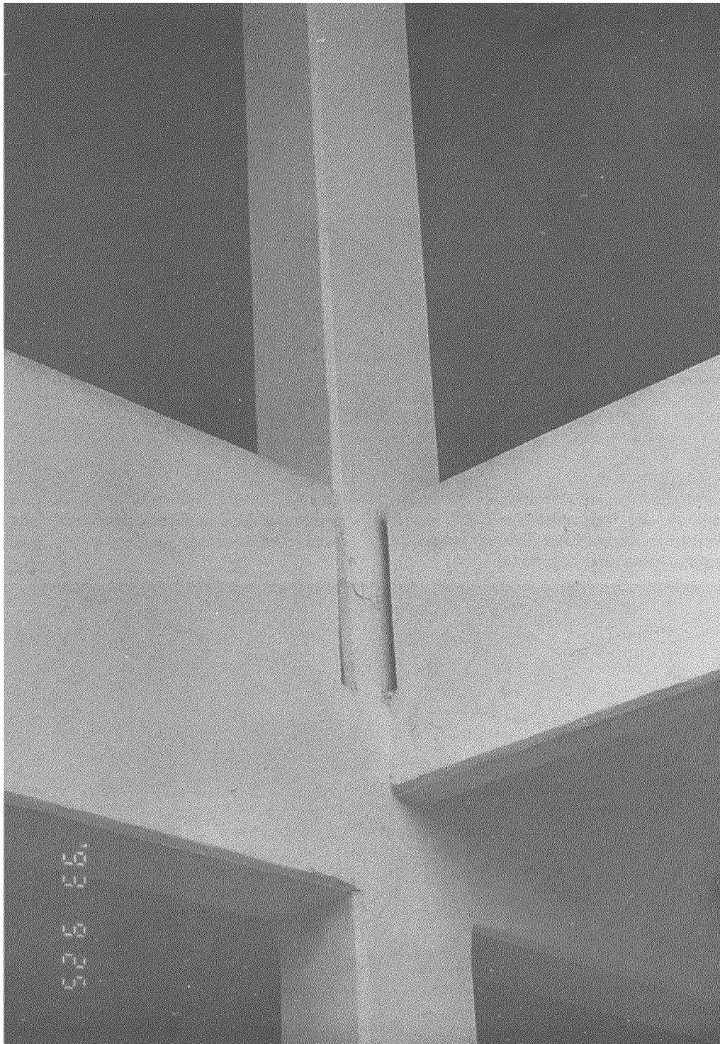
Foto 15.- Ranuras de separación entre los pretiles y las columnas de CR (septiembre de 1993)
