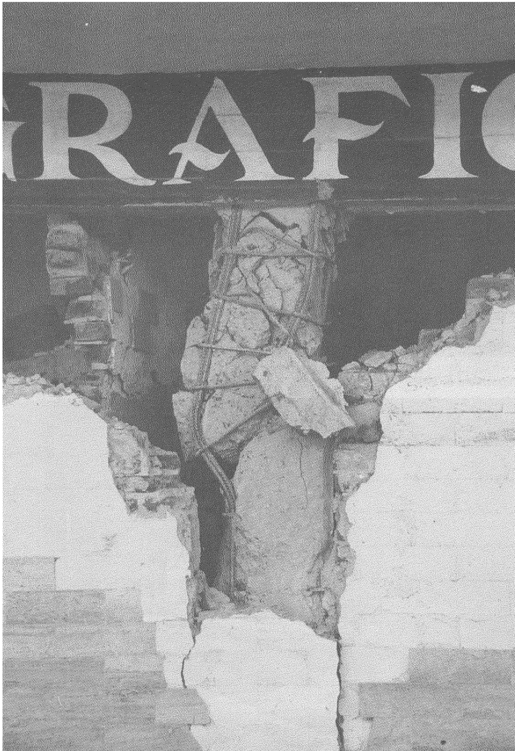
Foto 61.- Falla por cortante de la columna localizada en los ejes 1-C del plano de la Fig. 5 [1].
