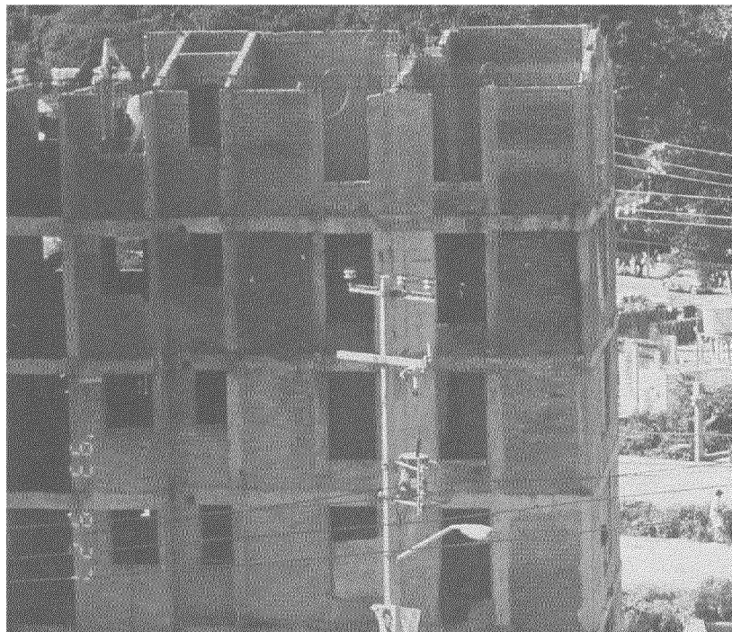
Foto 73 - Edificación de mampostería confinada en la cual parcialmente se emplean muros estructurales de concreto reforzado.
