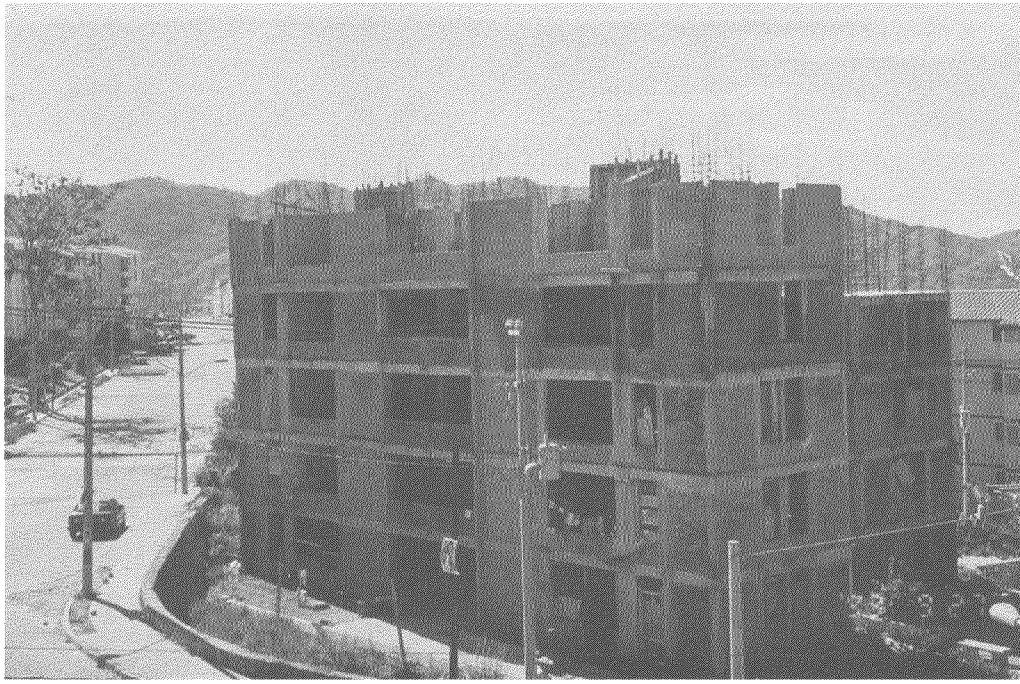
Foto 72.- Una edificación de mampostería con el proceso constructivo detenido.
