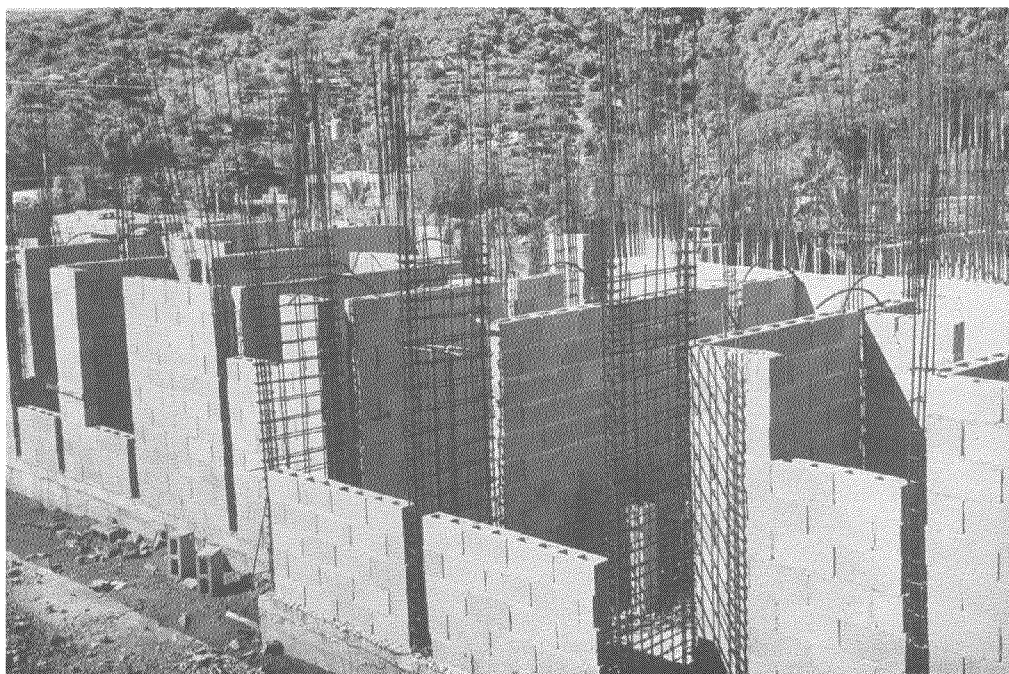
Foto 74.- Edificación de mampostería empleando bloque de concreto y muros estructurales de concreto reforzado.
