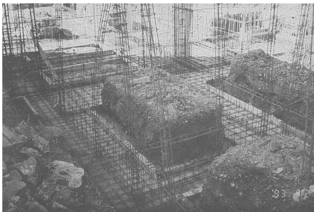
Foto 75.- Armado de la cimentación y de los muros de bloque de concreto y de concreto reforzado (1).
