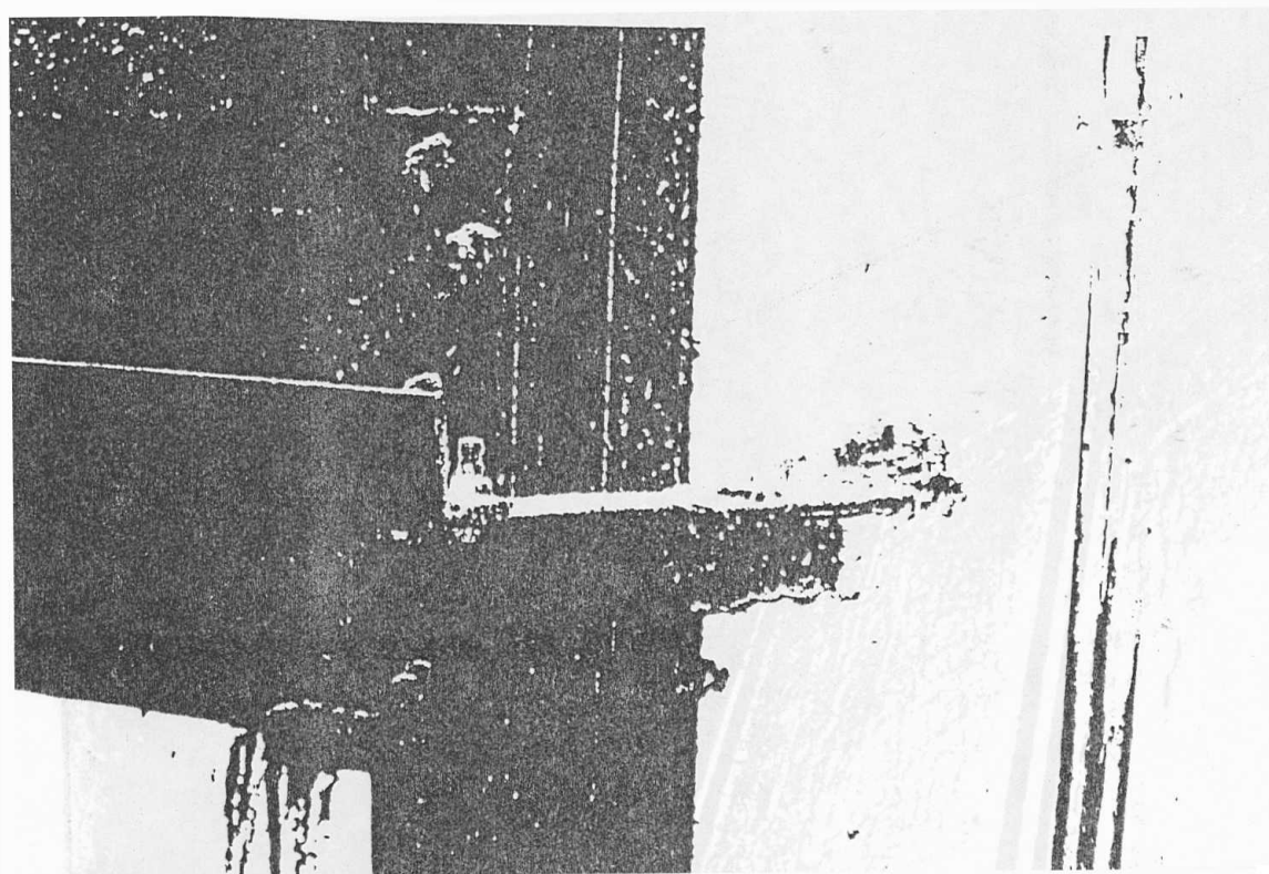
FIG. 4.44 DETALLE DEL SISTEMA GUIA DEL CONTRAPESO DEL ASCENSOR.
