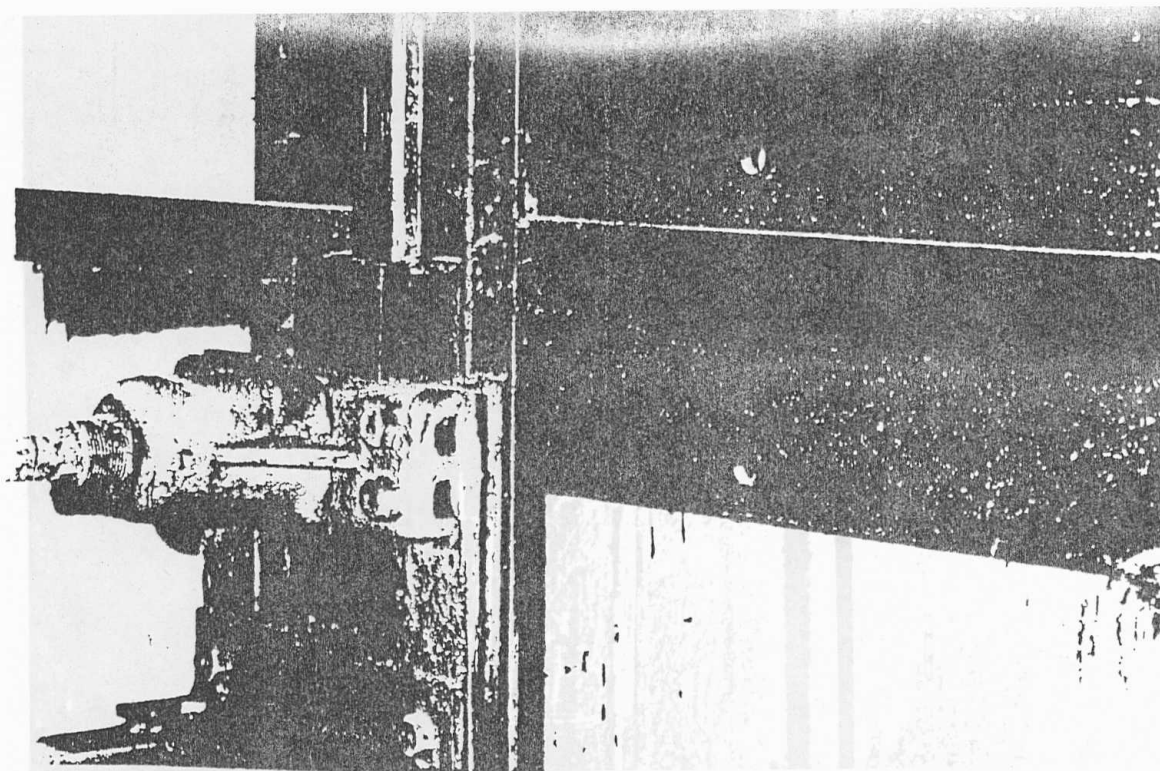
FIG. 4.43 DETALLE DEL SISTEMA GUIA DE LA CABINA DEL ASCENSOR.
