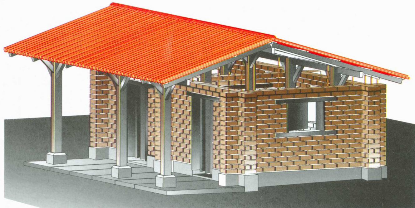
VISTA FRONTAL CON DETALLES
