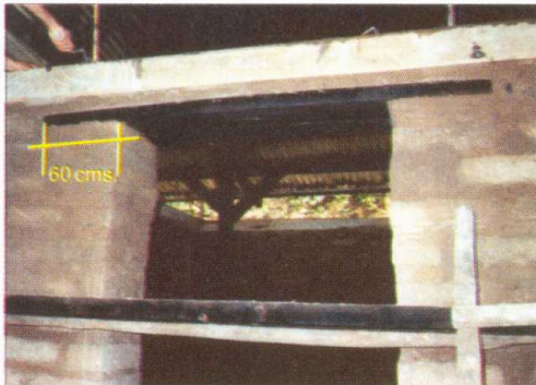
Cargadero de la puerta.
